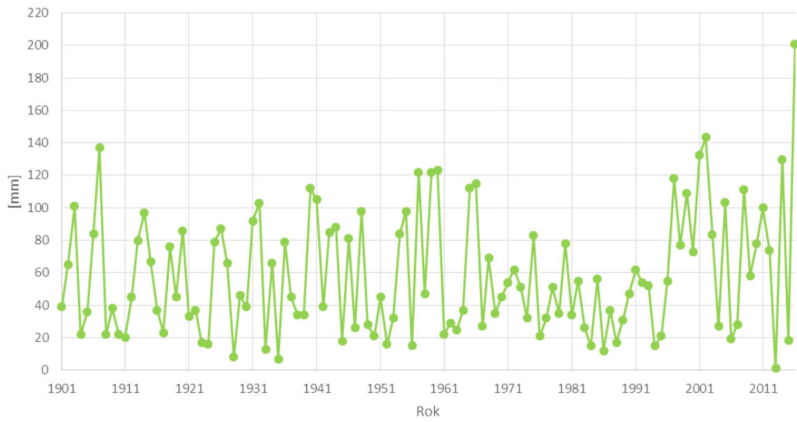
Mesačné úhrny zrážok v mesiaci júl na stanici Neded
