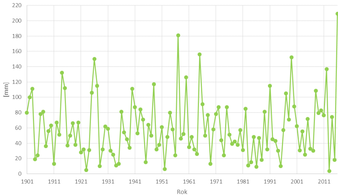
Mesačné úhrny zrážok v mesiaci júl na stanici Komárno - Hadovce
