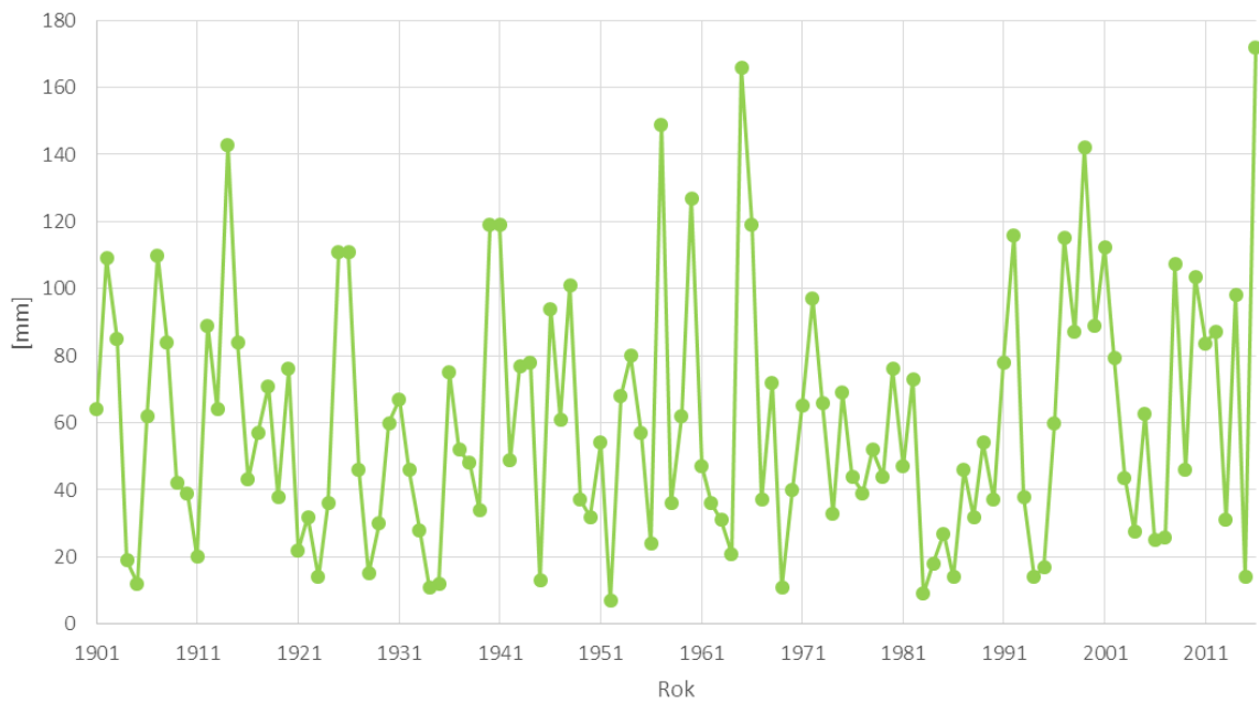
Mesačné úhrny zrážok v mesiaci júl na stanici Hurbanovo
