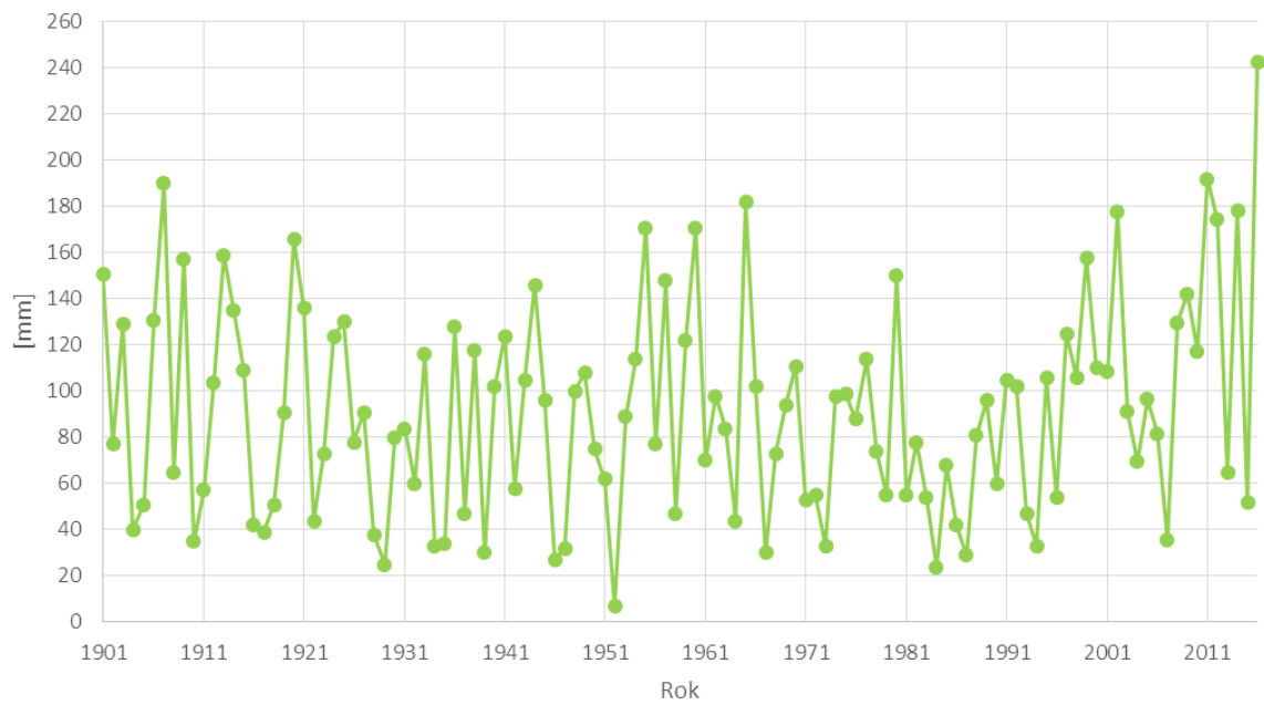
Mesačné úhrny zrážok v mesiaci júl na stanici Revúca
