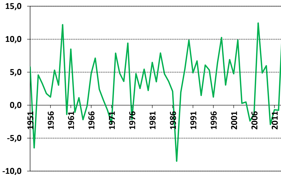
Priemerná denná teplota vzduchu v °C v Hurbanove pre 7. marec od roku 1951
