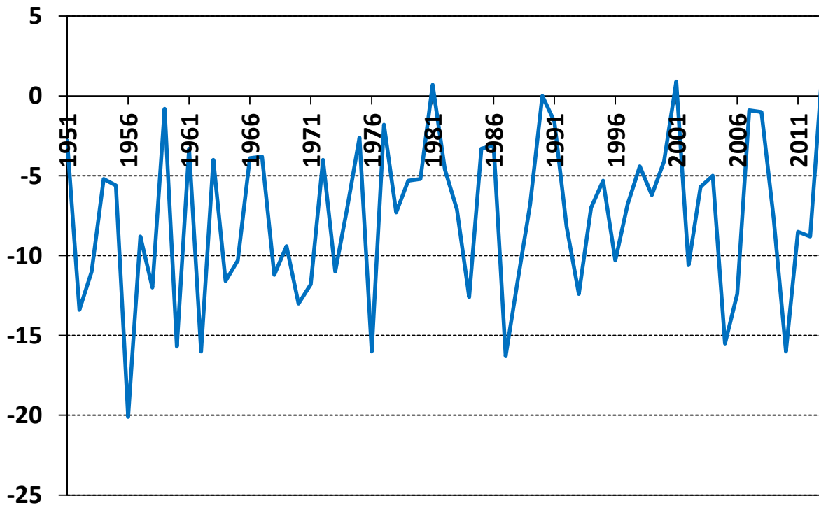
Maximálna denná teplota vzduchu v °C na Lomnickom štíte pre 8. marec od roku 1951
