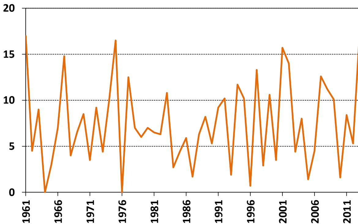
Maximálna denná teplota vzduchu v °C v Somotore pre 11. marec od roku 1961
