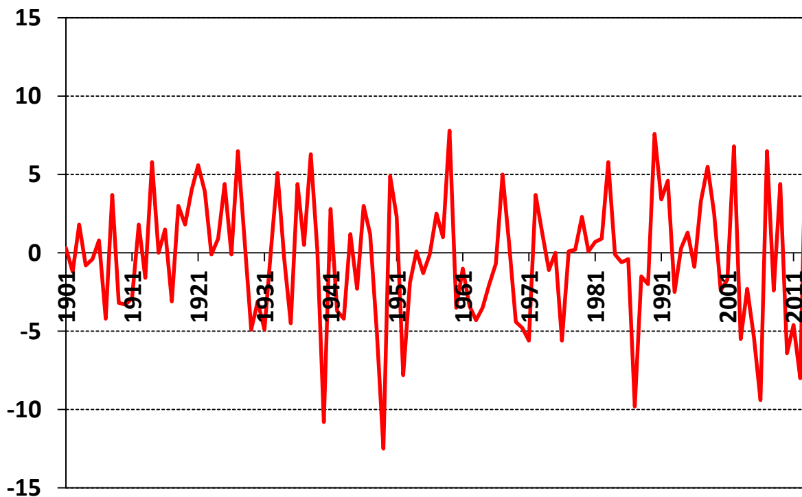
Minimálna denná teplota vzduchu v °C v Hurbanove pre 7. marec od roku 1901
