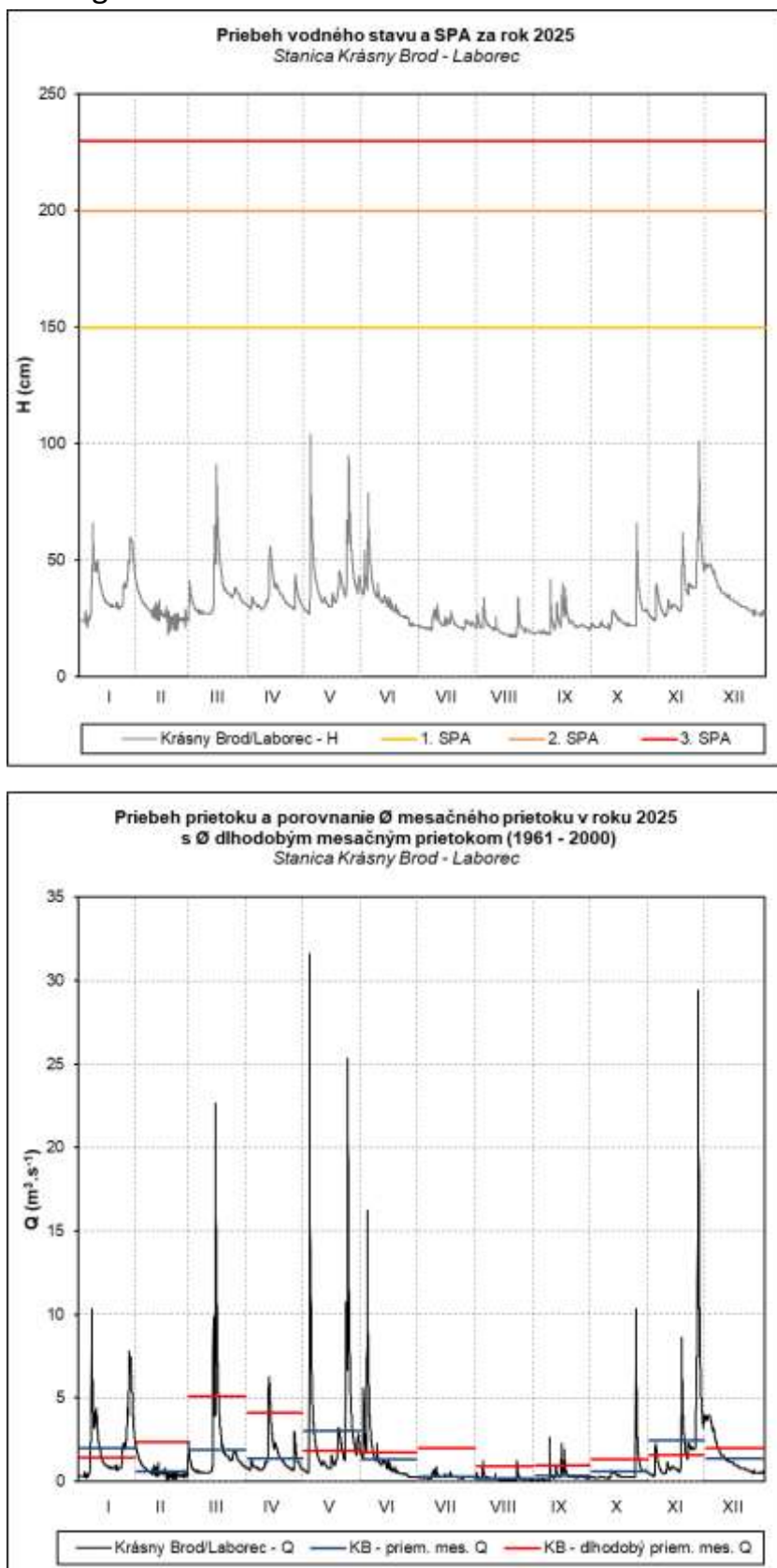
Obr. 61 Priebek vodného stavu a prietoku v stanici Krásny Brod – Laborec
