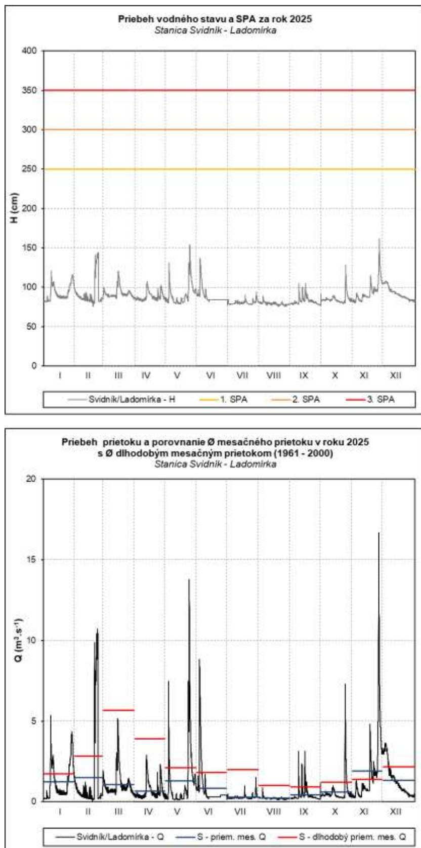
Obr. 71 Priebeh vodného stavu a prietoku v stanici Svidník – Ladomírka
