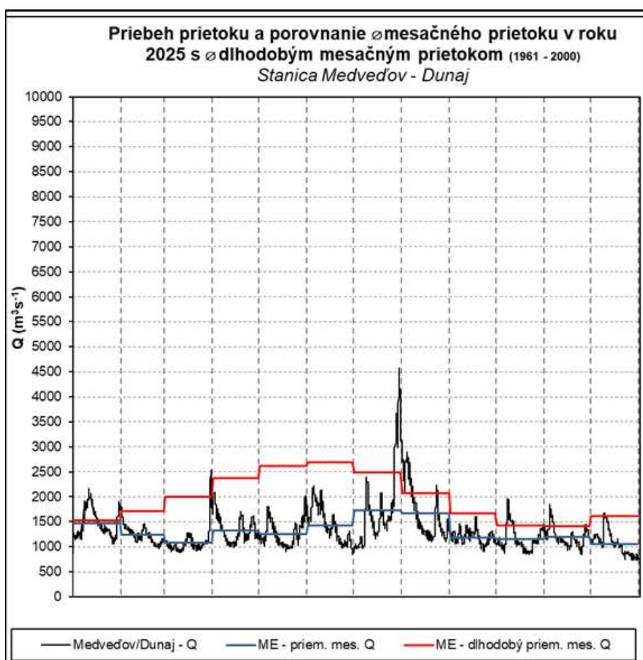
Obr. 5 Priebeh vodného stavu a prietoku v stanici Medveďov – Dunaj
