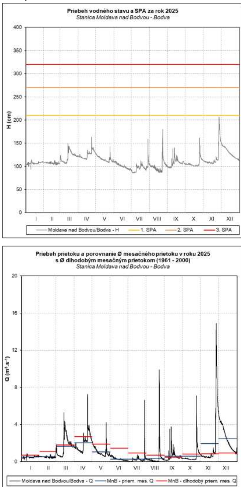
Obr. 50 Priebek vodného stavu a prietoku v stanici Moldava nad Bodvou – Bodva
