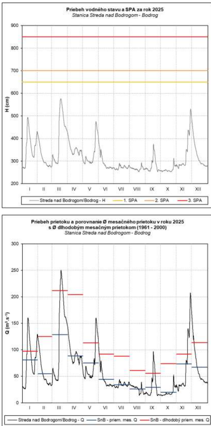
Obr. 74 Priebeh vodného stavu a prietoku v stanici Streda nad Bodrogom – Bodrog
