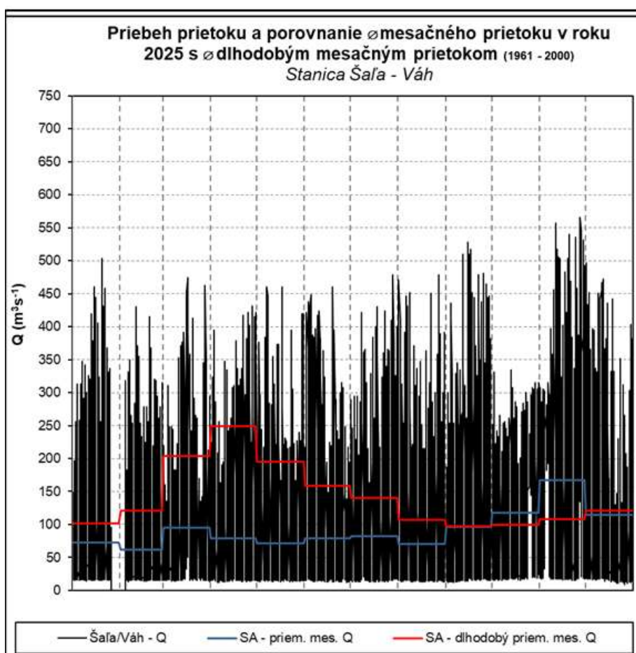
Obr. 26 Priebeh vodného stavu a prietoku v stanici Šaľa – Váh
