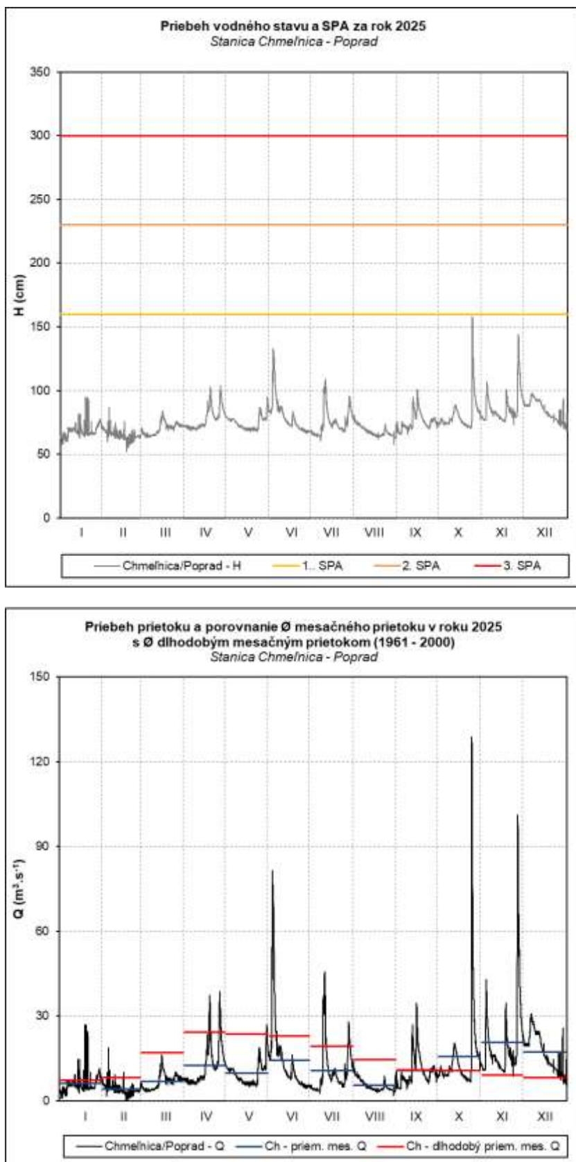
Obr. 76 Priebeh vodného stavu a prietoku v stanici Chmeľnica – Poprad
