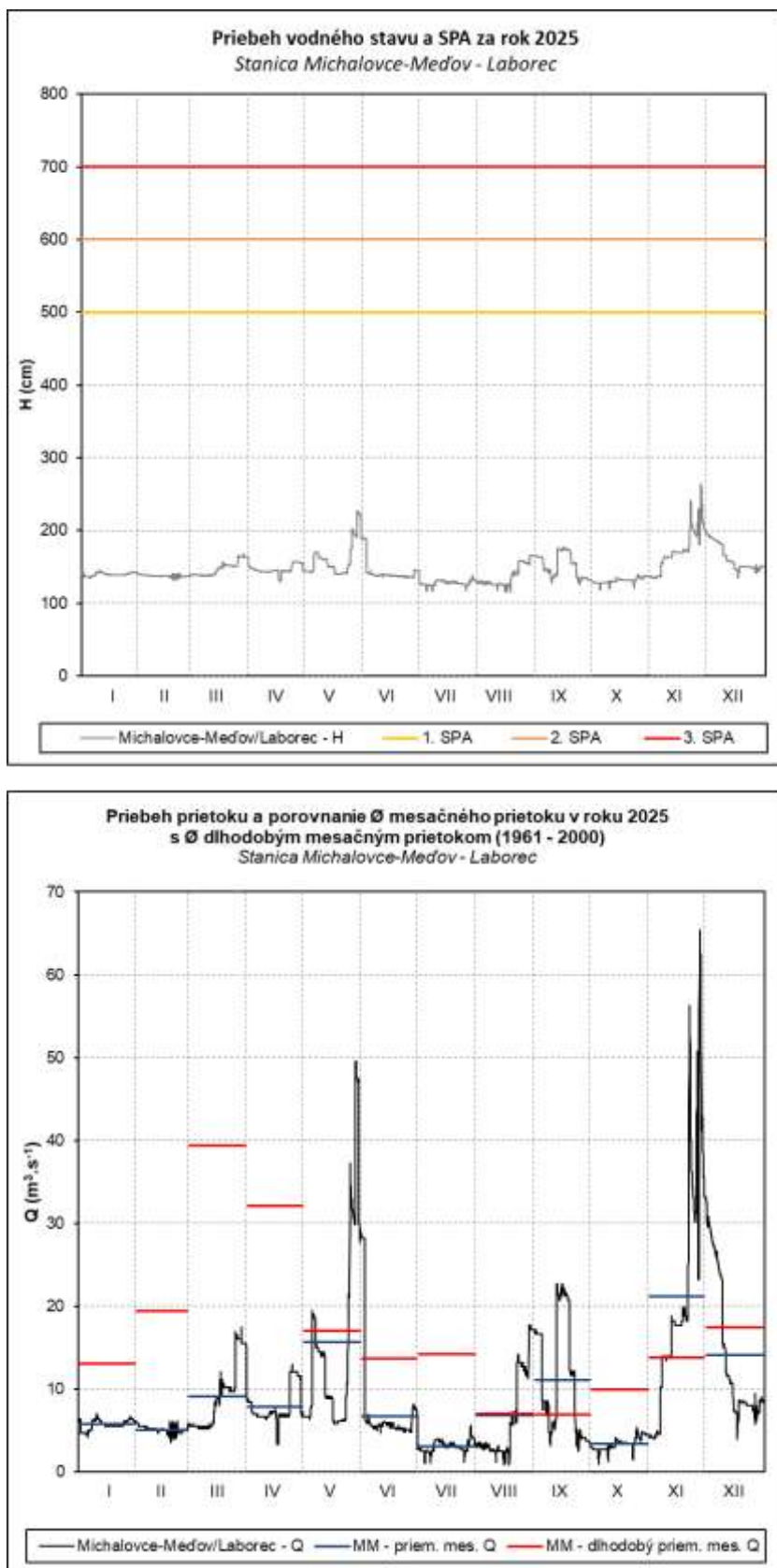
Obr. 64 Priebeh vodného stavu a prietoku v stanici Michalovce-Meďov – Laborec
