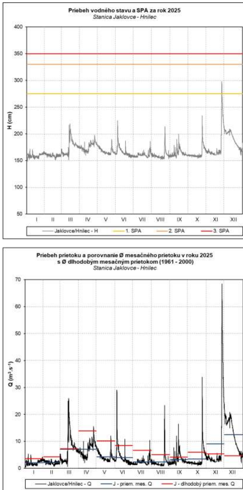
Obr. 55 Priebeh vodného stavu a prietoku v stanici Jaklovce – Hnilec
