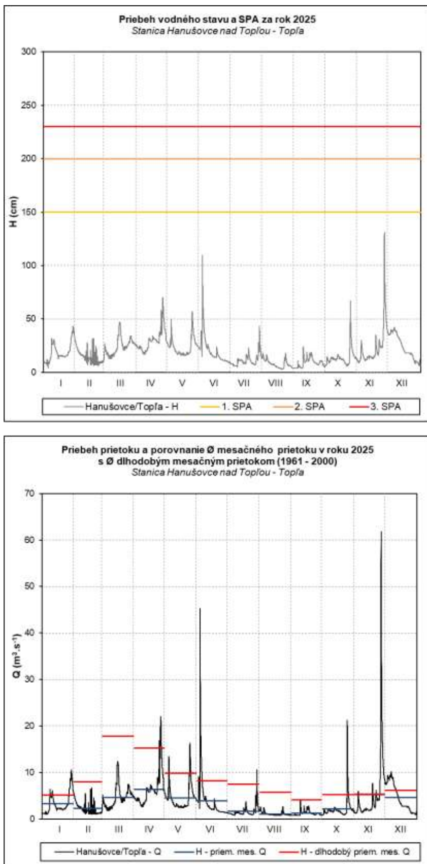
Obr. 69 Priebeh vodného stavu a prietoku v stanici Hanušovce nad Topľou – Topľa
