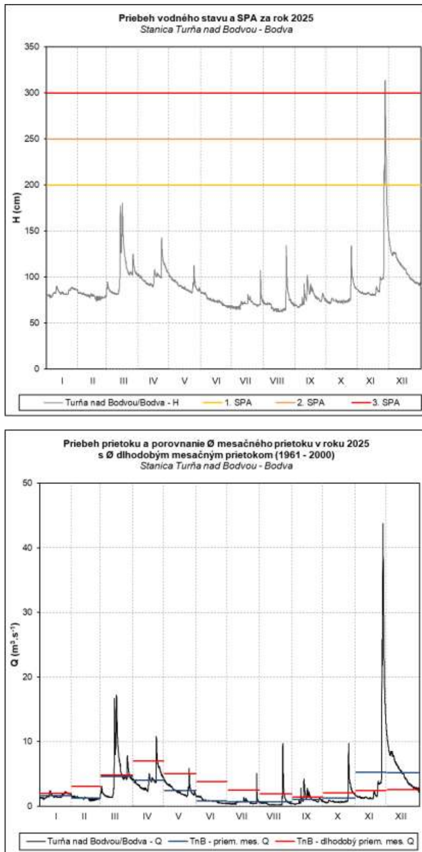
Obr. 51 Priebeh vodného stavu a prietoku v stanici Turňa nad Bodvou – Bodva
