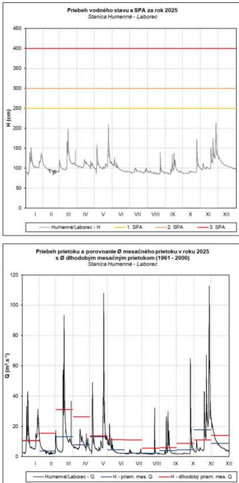
Obr. 63 Priebeh vodného stavu a prietoku v stanici Humenné – Laborec
