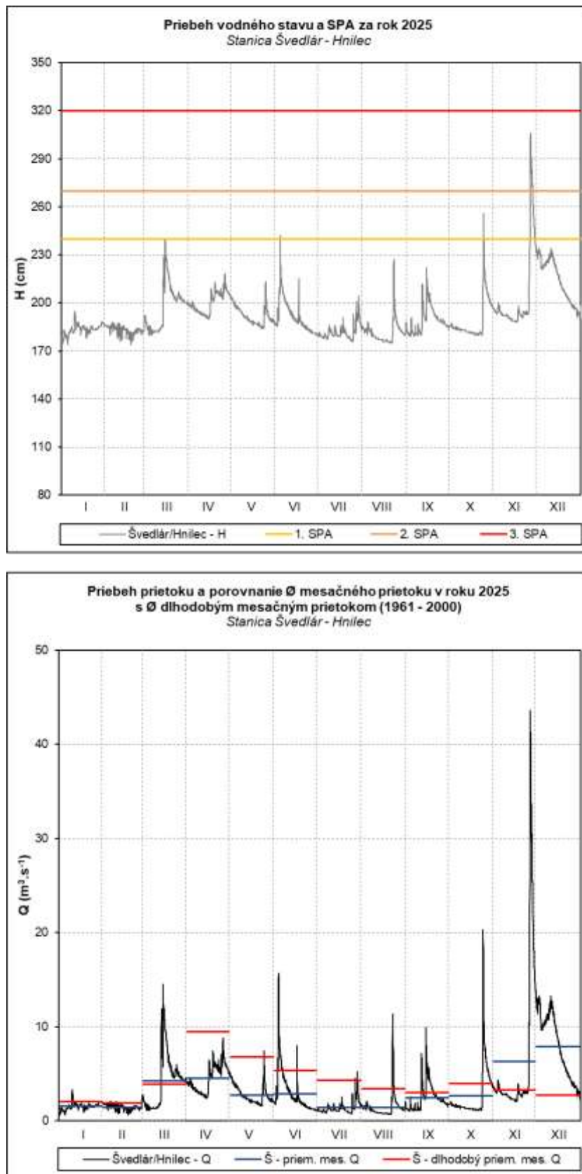
Obr. 54 Priebek vodného stavu a prietoku v stanici Švedlár – Hnilec
