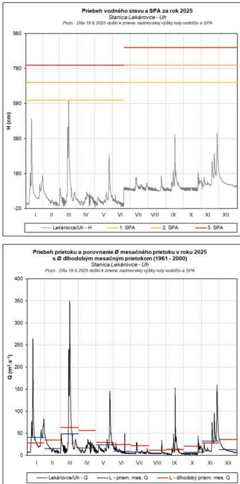
Obr. 65 Priebeh vodného stavu a prietoku v stanici Lekárovce – Uh
