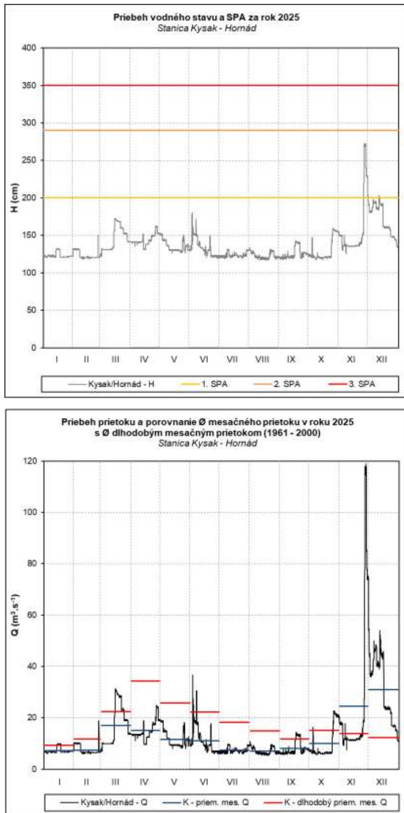
Obr. 56 Priebeh vodného stavu a prietoku v stanici Kysak – Hornád
