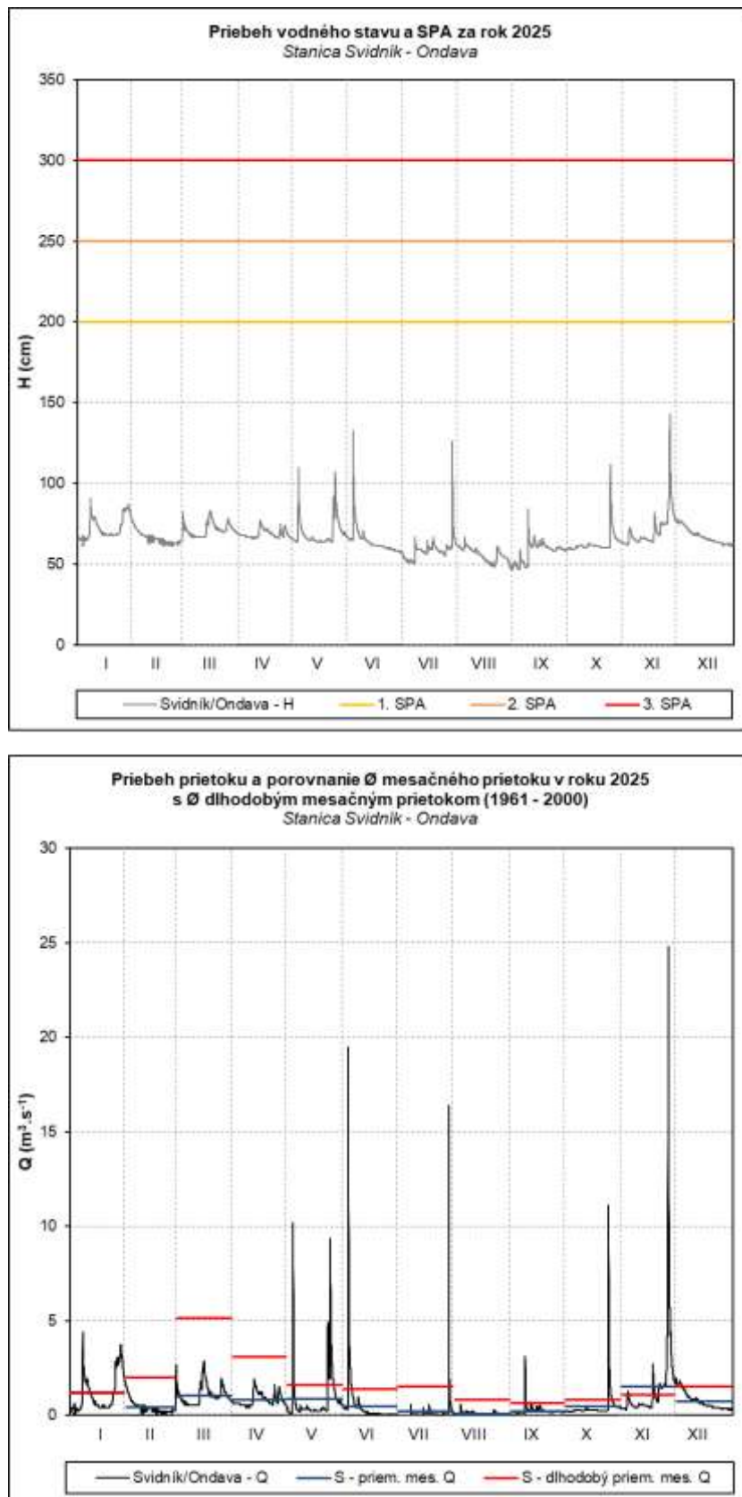
Obr. 70 Priebeh vodného stavu a prietoku v stanici Svidník – Ondava
