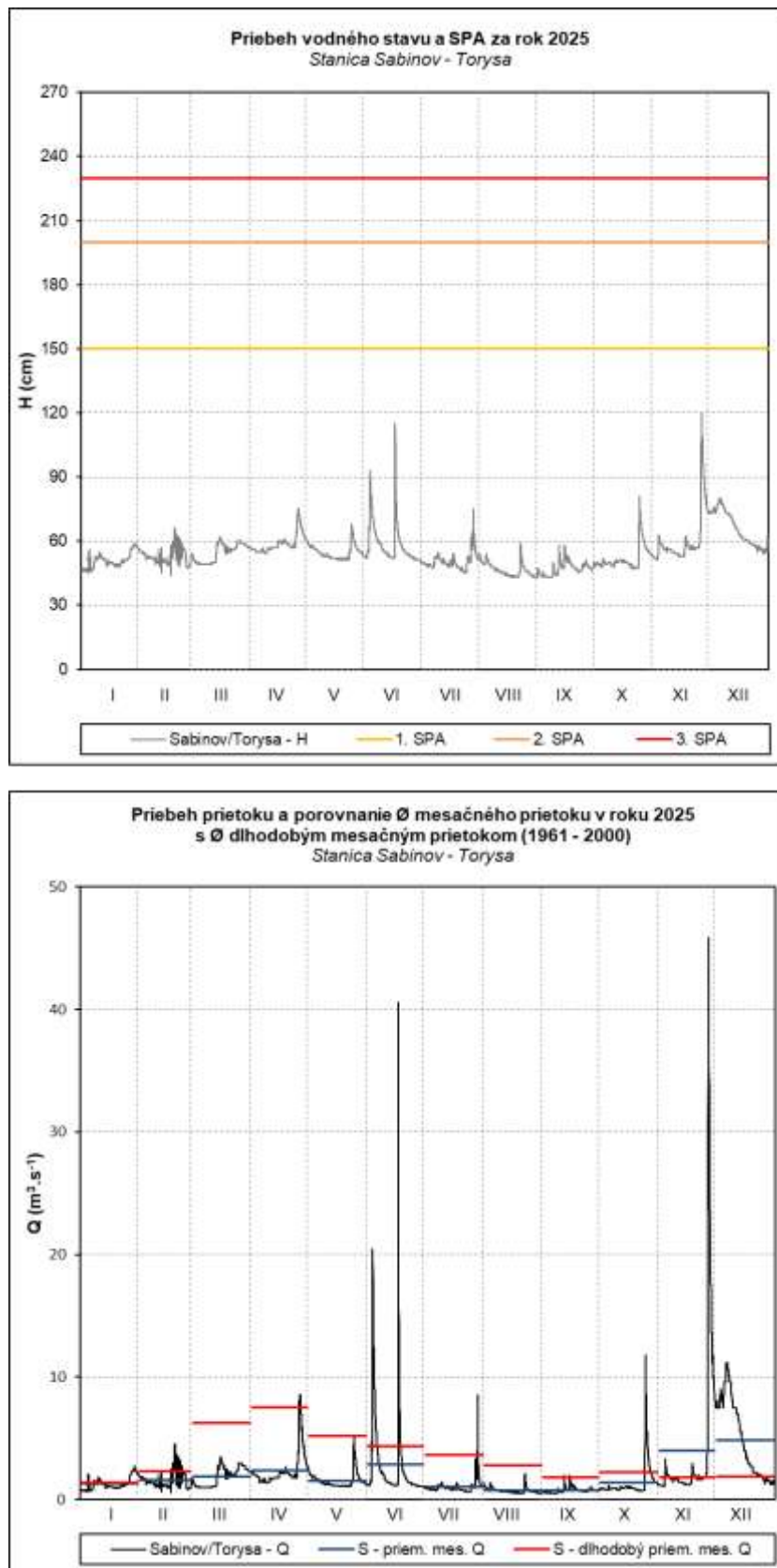
Obr. 57 Priebeh vodného stavu a prietoku v stanici Sabinov – Torysa
