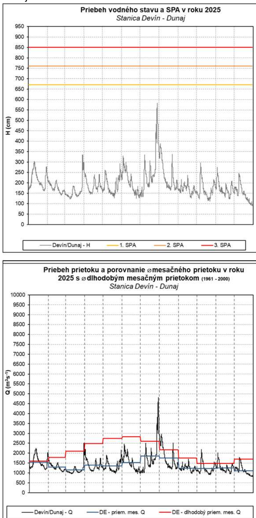
Obr. 3 Priebeh vodného stavu a prietoku v stanici Devín – Dunaj
