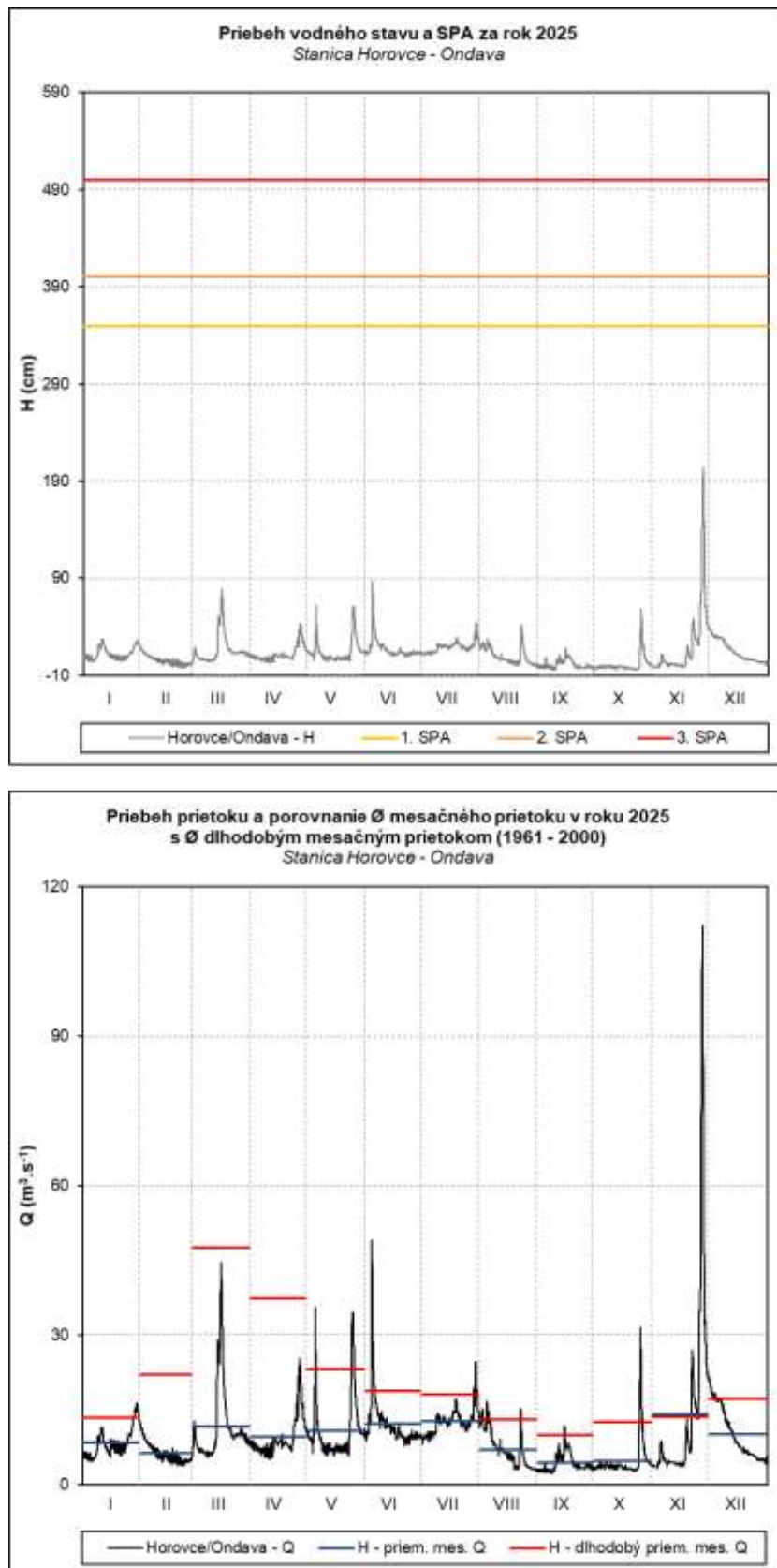
Obr. 73 Priebeh vodného stavu a prietoku v stanici Horovce – Ondava
