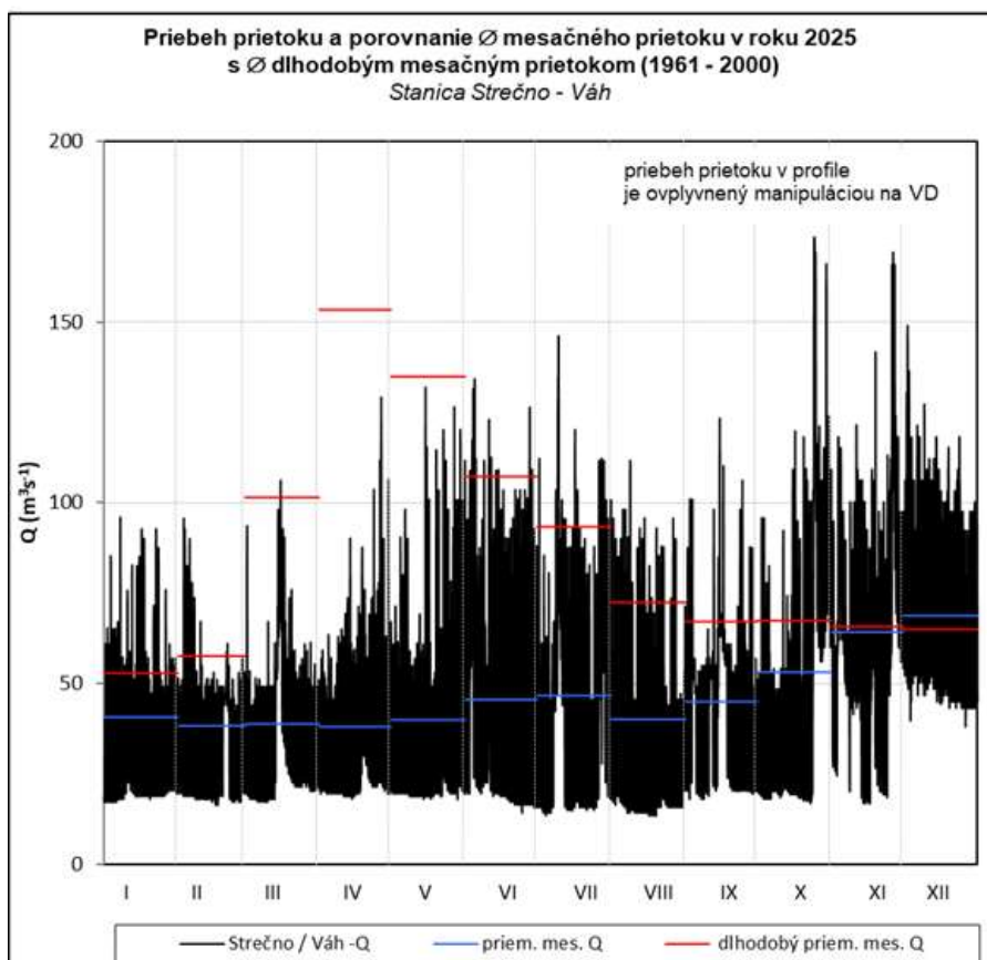
Obr. 18 Priebeh vodného stavu a prietoku v stanici Strečno – Váh
