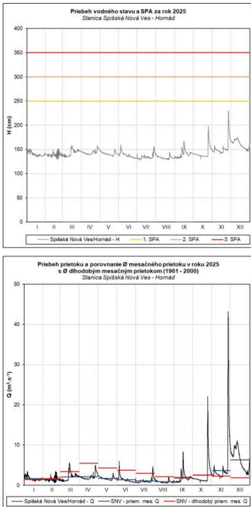
Obr. 52 Priebek vodného stavu a prietoku v stanici Spišská Nová Ves – Hornád
