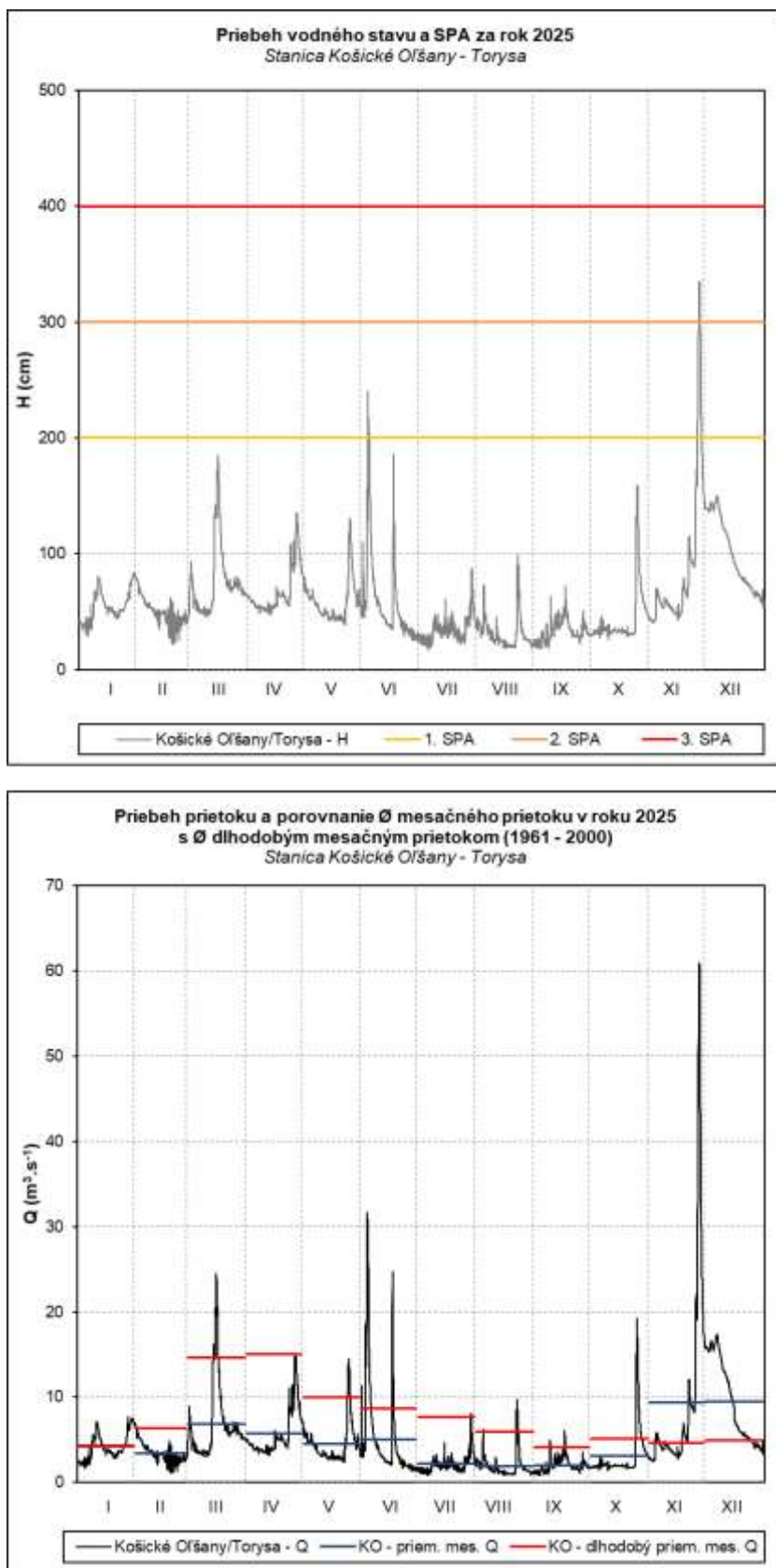
Obr. 59 Priebeh vodného stavu a prietoku v stanici Košické Oľšany – Torysa
