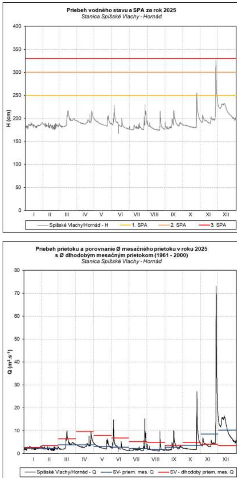
Obr. 53 Priebeh vodného stavu a prietoku v stanici Spišské Vlachy – Hornád
