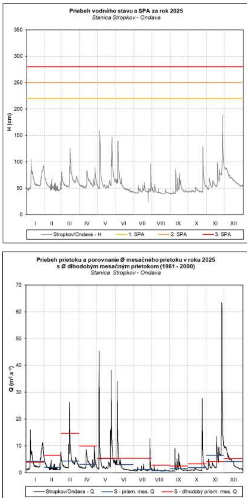
Obr. 72 Priebeh vodného stavu a prietoku v stanici Stropkov – Ondava
