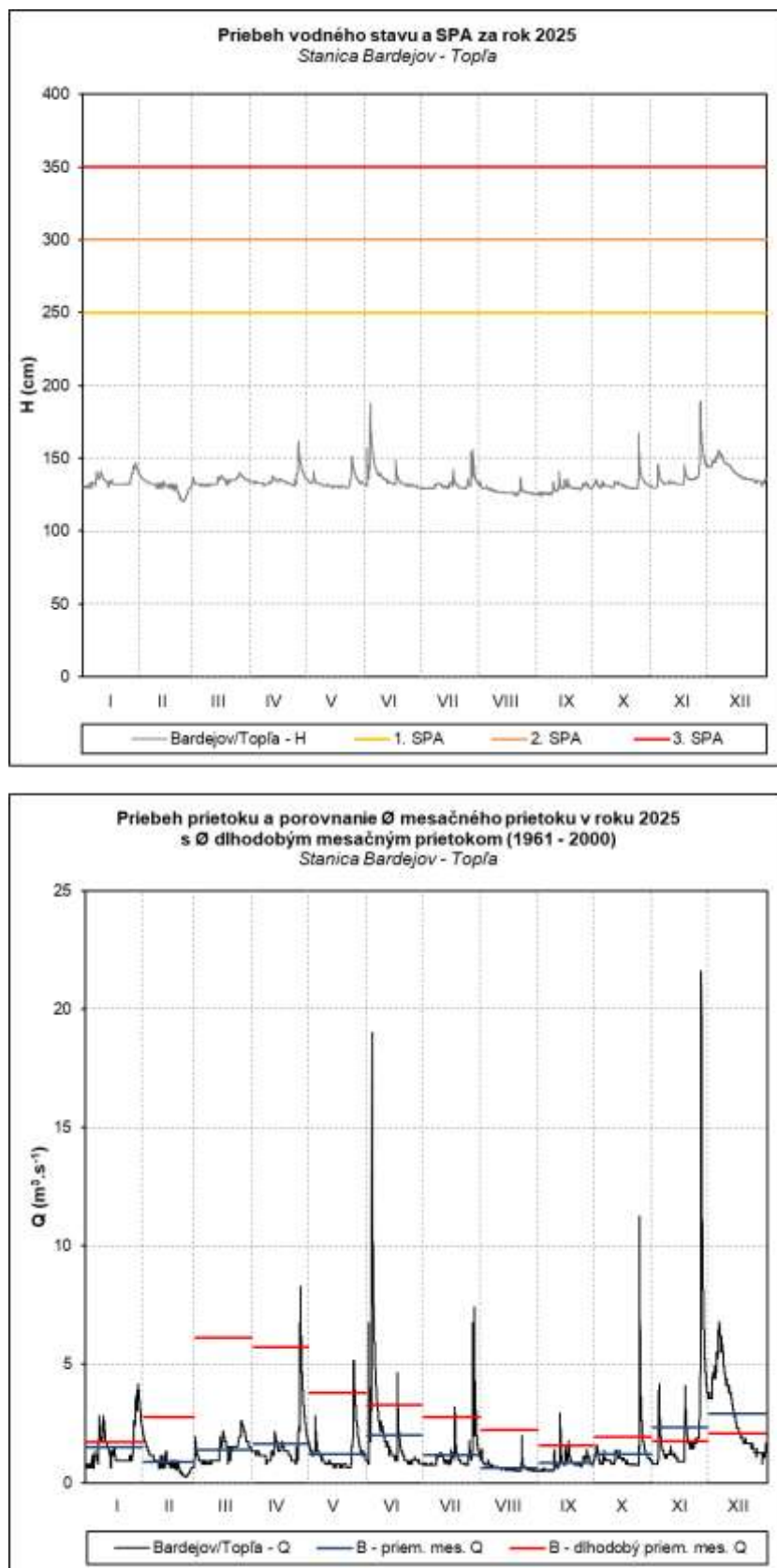
Obr. 68 Priebeh vodného stavu a prietoku v stanici Bardejov – Topľa
