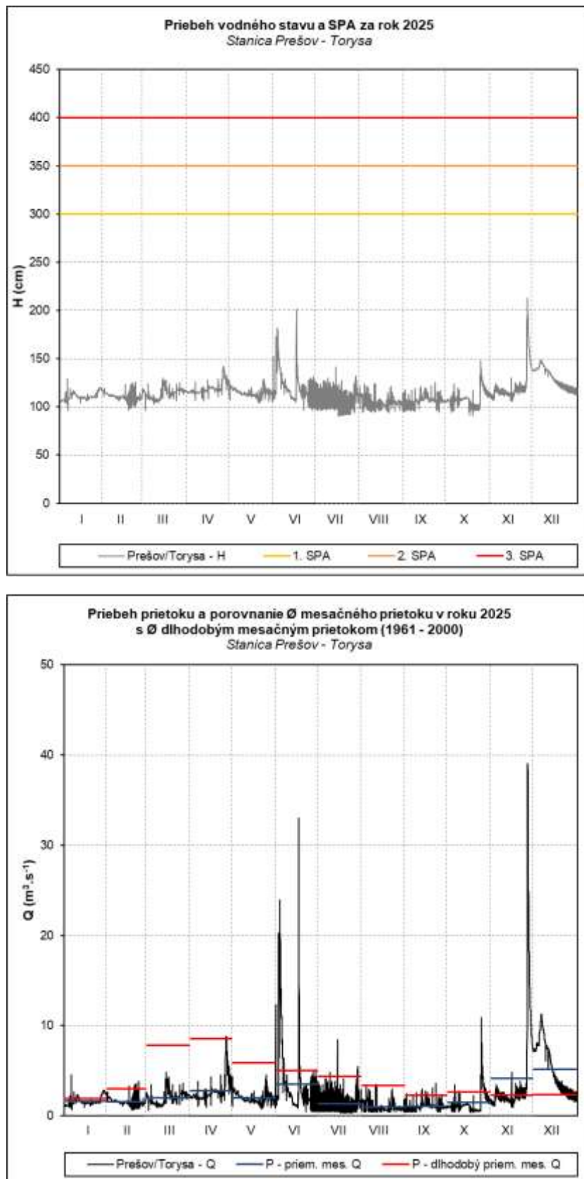
Obr. 58 Priebeh vodného stavu a prietoku v stanici Prešov – Torysa
