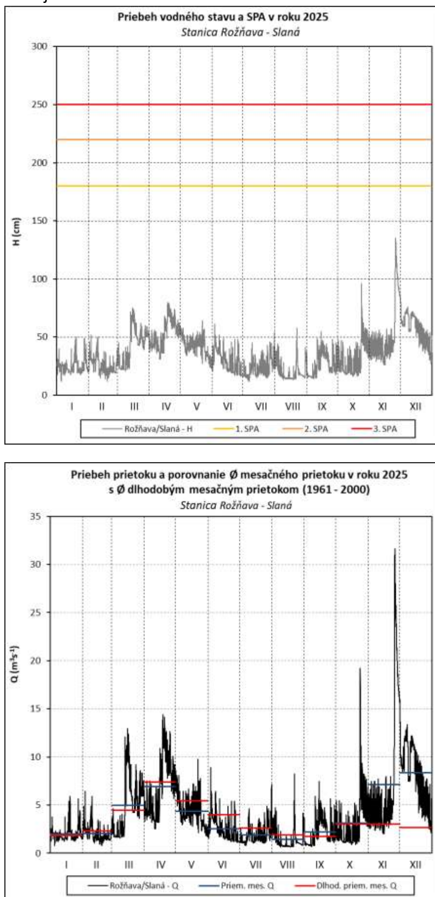
Obr. 43 Priebek vodného stavu a prietoku v stanici Rožňava – Slaná
