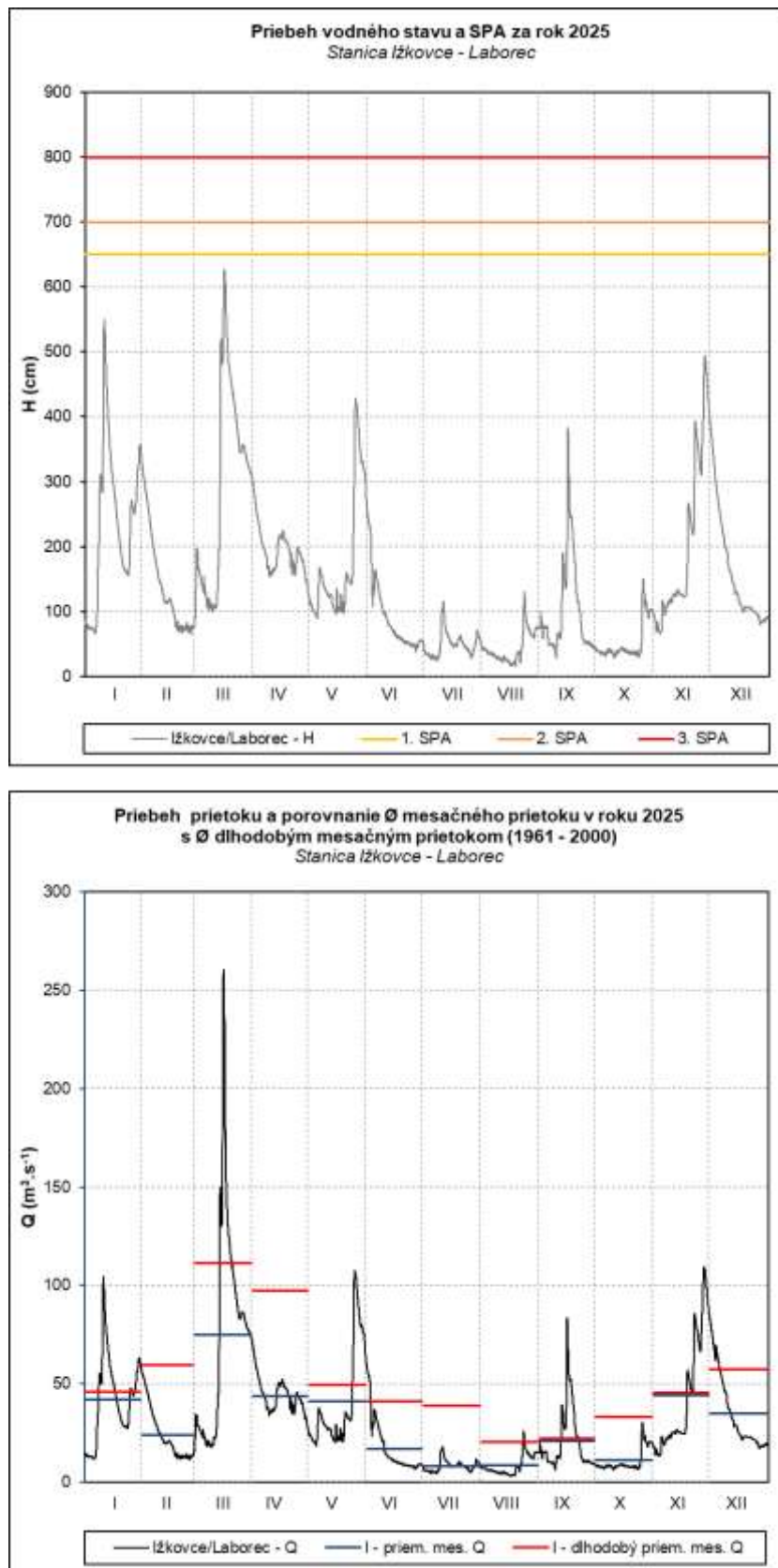
Obr. 66 Priebeh vodného stavu a prietoku v stanici Ižkovce – Laborec
