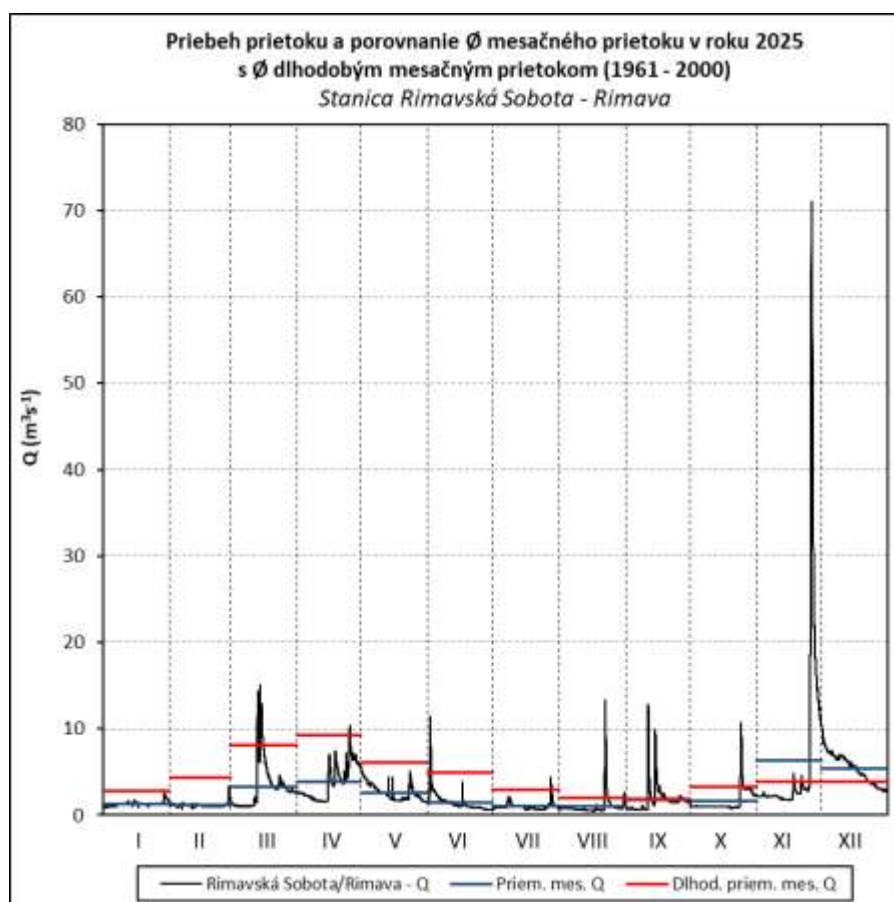
Obr. 48 Priebeh vodného stavu a prietoku v stanici Rimavská Sobota-Sobôtka – Rimava
