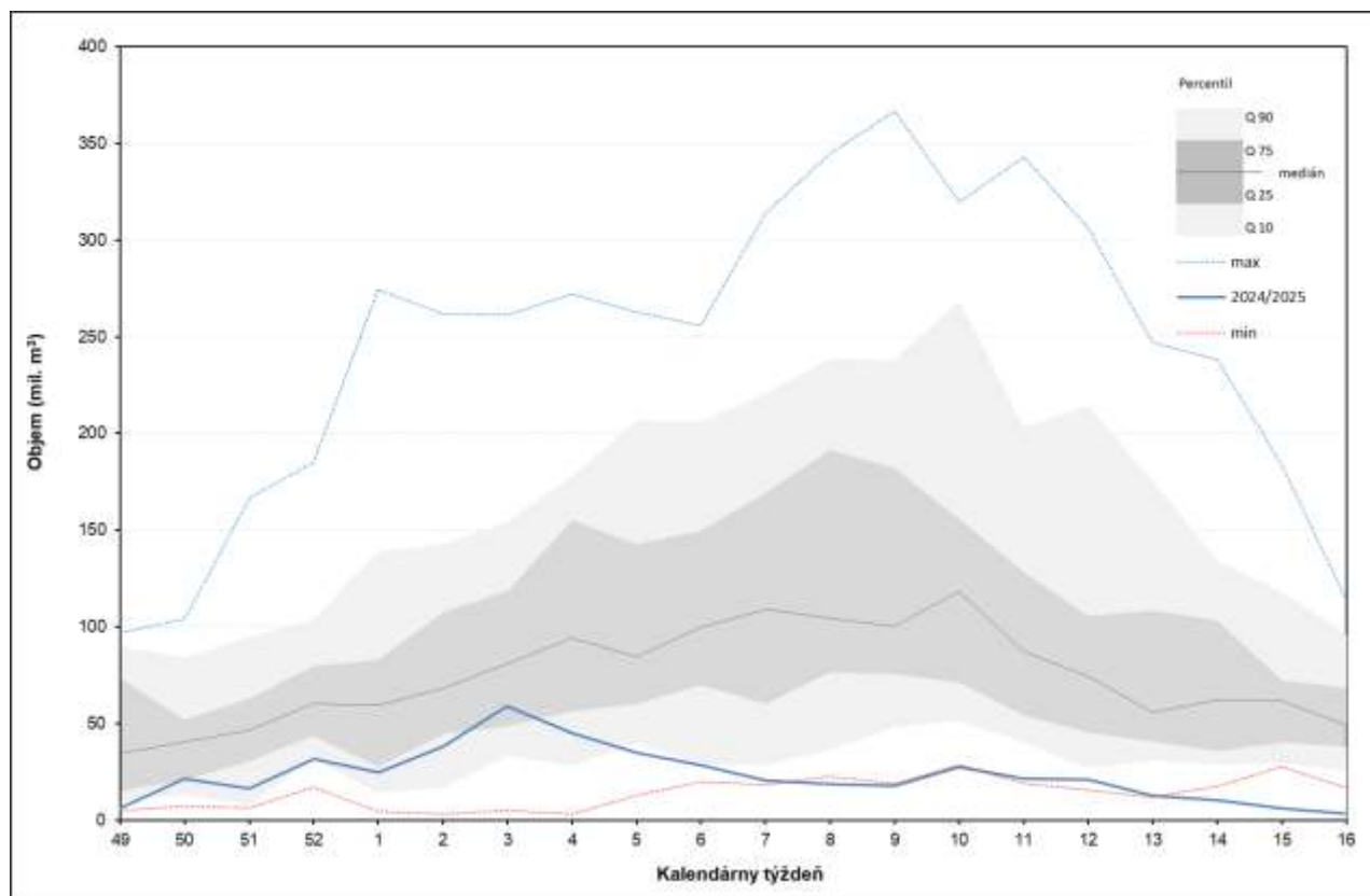
Obr. 5.3.3 Pribeh celkových zásob vody v snehovej pokrývke (mil. m 3 ) v povodí „nášov“ počas zimy 2024/2025 v štatistickom porovnaní so zimami za normálové obdobie 1991 – 2020
