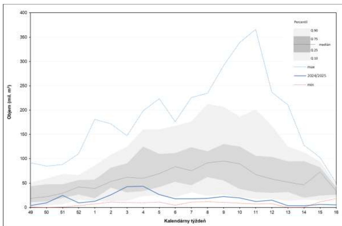
Obr. 5.4.3 Priebeh celkových zásob vody v snehovej pokrývke (mil. m 3 ) v povodí Popradu počas zimy 2024/2025 v štatistickom porovnaní so zimami za normálové obdobie 1991 – 2020
