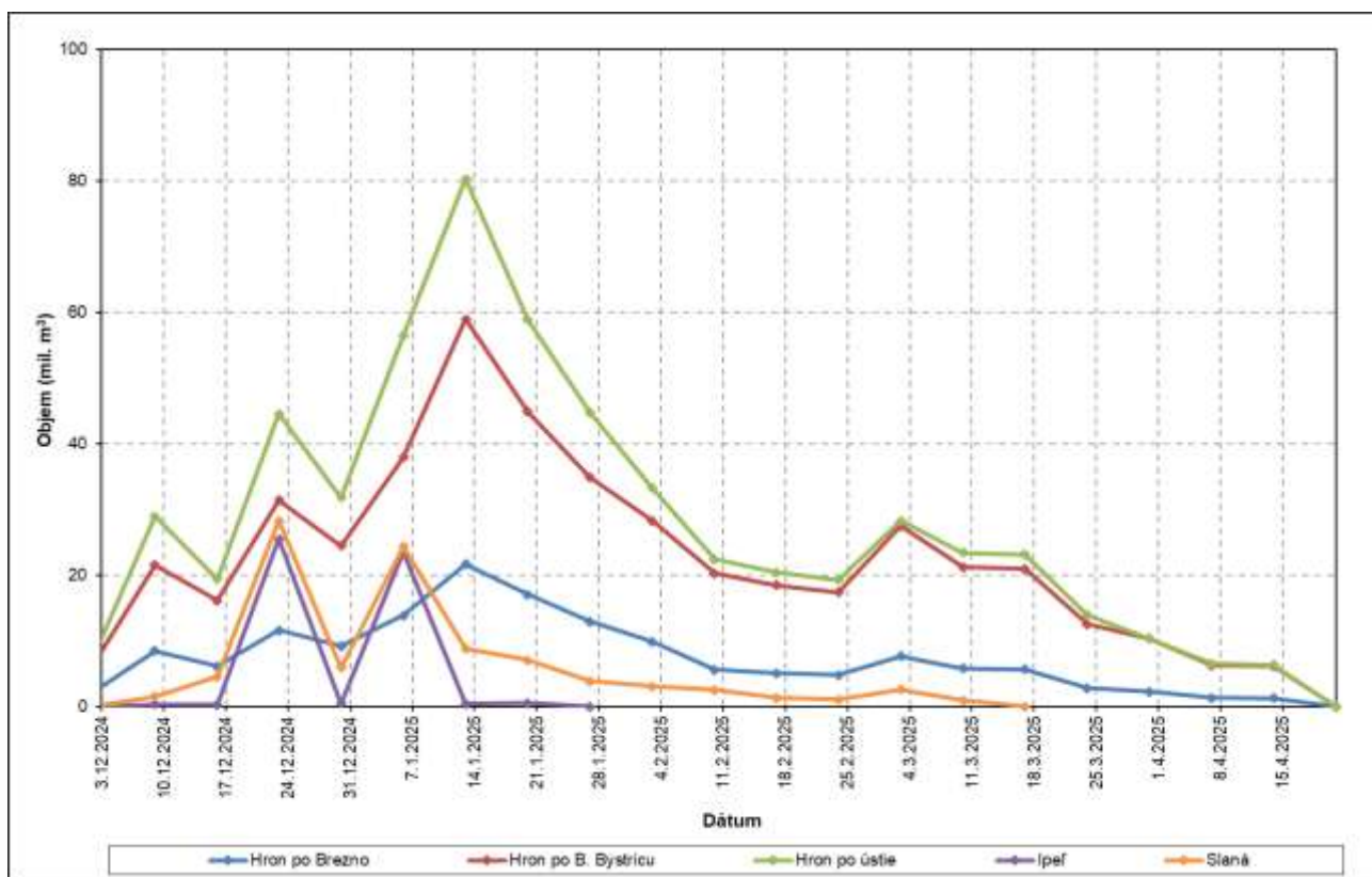
Obr. 5.3.1 Pribeh zásob vody v snehovej pokrývke v povodiach Hrona, Ipľa a Slanej v zime 2024/2025
