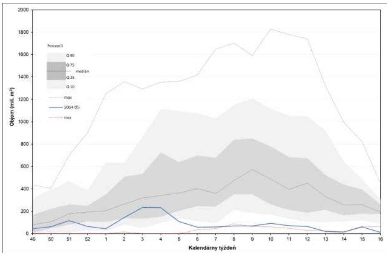
Obr. 5.2.3 Priebieh celkových zásob vody v snehovej pokrývke (mil. m 3 ) v povodí Váhu po profil VD Nosice počas zimy 2024/2025 v štatistickom porovnaní so zimami za normálové obdobie 1991 – 2020
