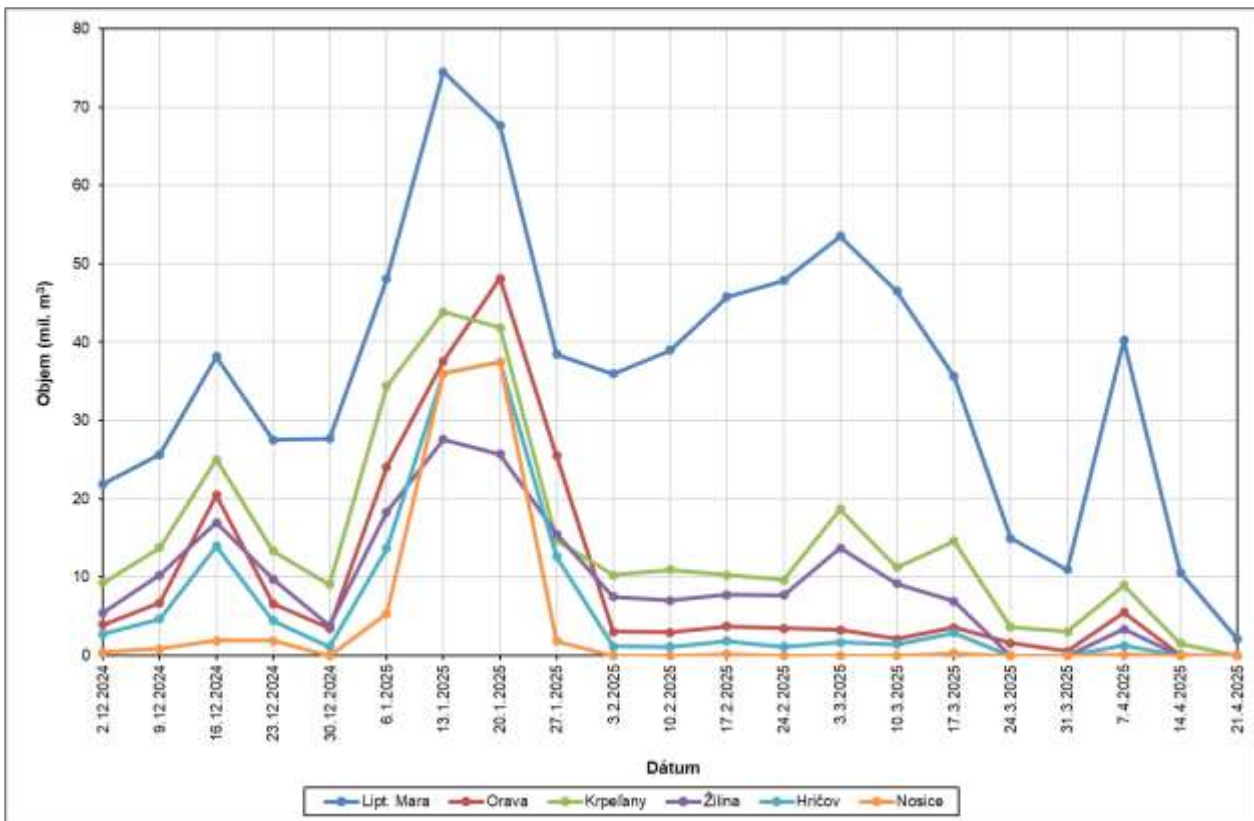
Obr. 5.2.1 Priebek zásob vody v snehovej pokrývke (mil. m 3 ) k vybraným vodným dielam v povodí Váhu počas zimy 2024/2025
