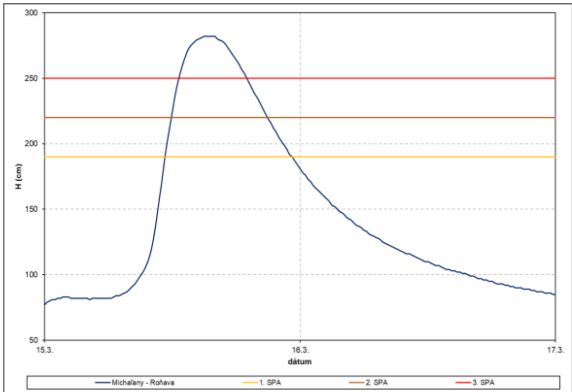
Obr. 4.10.2 Priebeh vodnej hladiny vo vodomernej stanici Michalany – Roňava, marec 2025
