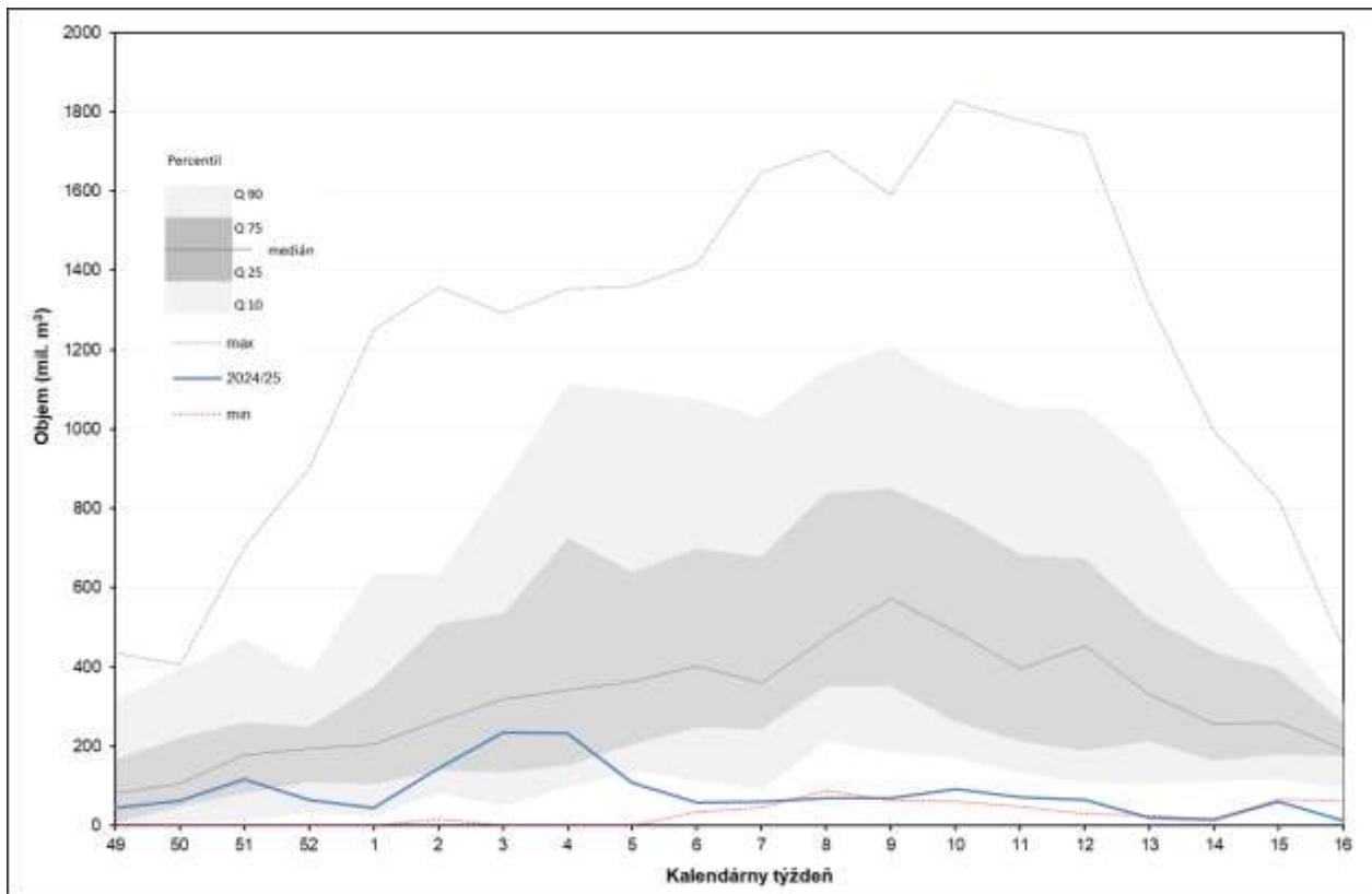
Obr. 5.2.3 Priebeh celkových zásob vody v snehovej pokrývke (mil. m 3 ) v povodí Váhu po profil VD Nosice počas zimy 2024/2025 v štatistickom porovnaní so zimami za normálové obdobie 1991 – 2020
