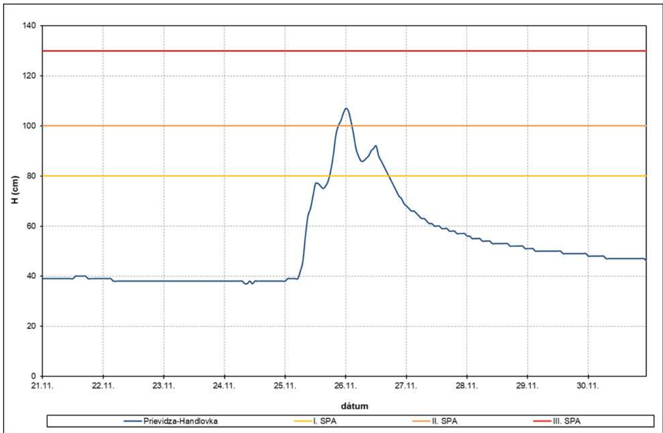
Obr. 4.4.14 Priebek vodnej hladiny vo vodomernej stanici Prievidza - Handlovka, november 2025
