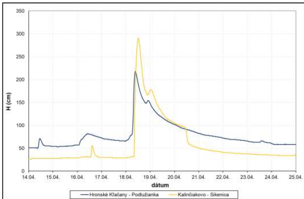
Obr. 4.5.4 Priebeh vodných hladín na tokoch v povodí dolného Hrona, apríl 2025
