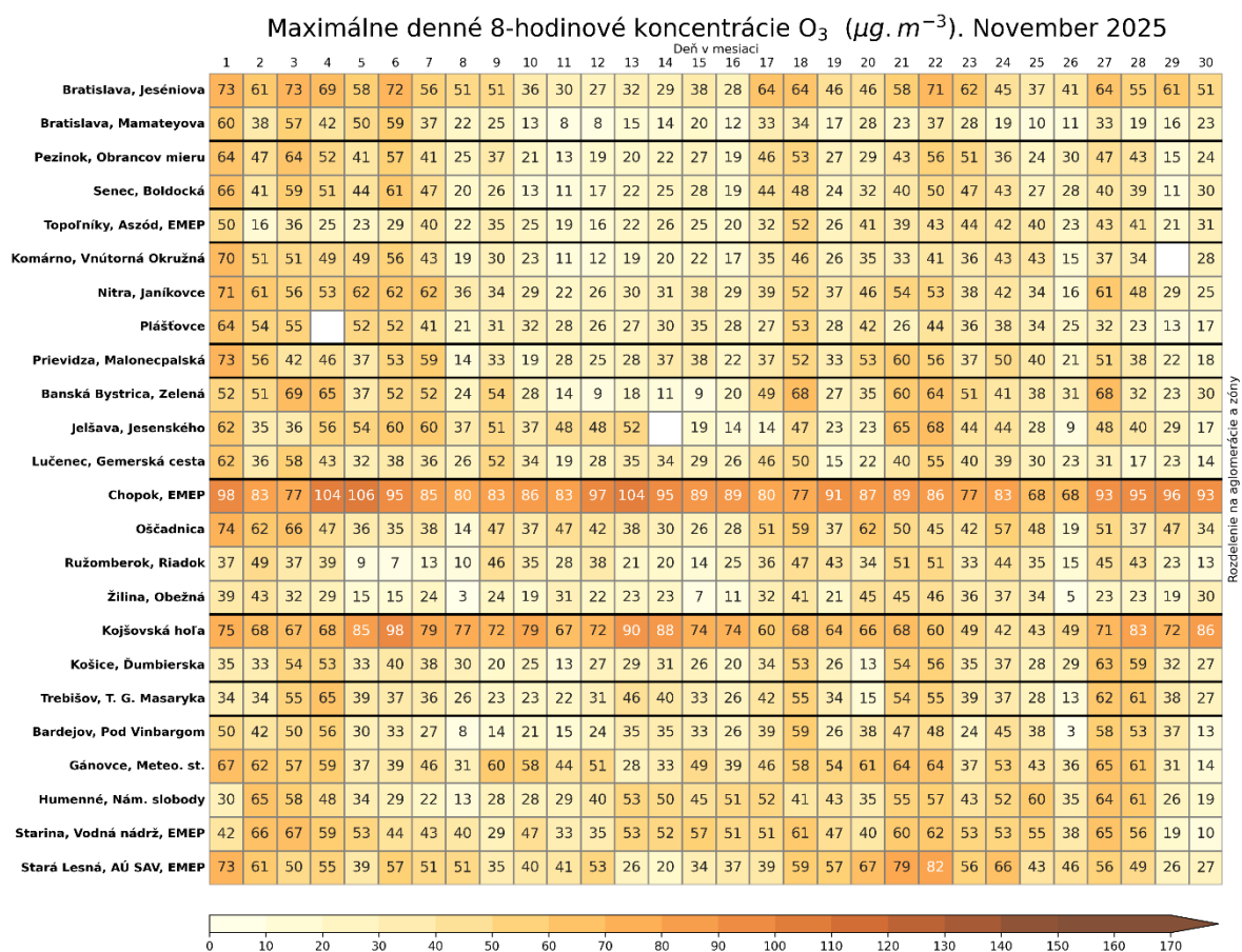
Obr. 5 Maximálne denné 8-hodinové koncentrácie O 3 namerané v sieti NMSKO.
