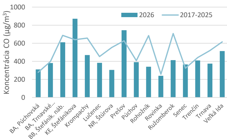
Obr. 8 Mesačné koncentrácie ( \mu\text{g}/\text{m}^3 ) CO v porovnaní z referenčným obdobím
