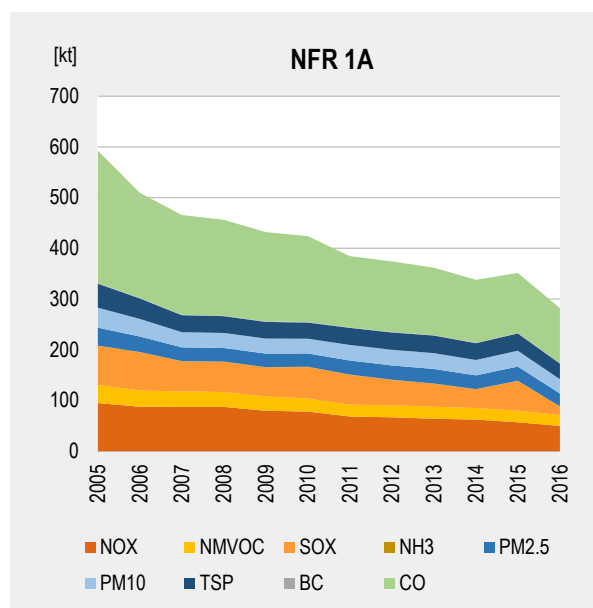
Obr. 5.6 Vývojové trendy emisií znečisťujúcich látok v sektore energetika a činnosti súvisiace so spaľovaním palív v rokoch 2005 – 2016
