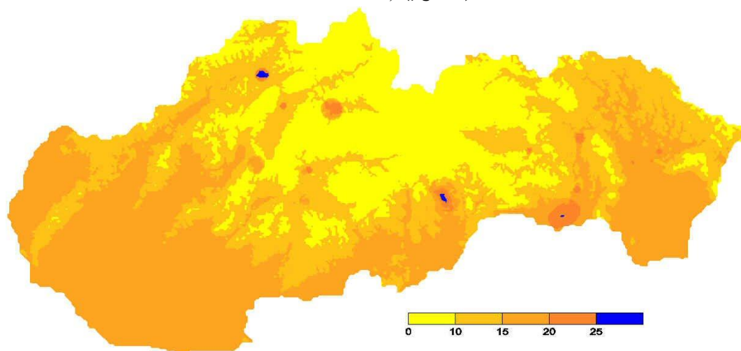
Obr. 4.14 Priemerná ročná koncentrácia PM_{2.5} ( \mu g \cdot m^{-3} ), rok 2017.
