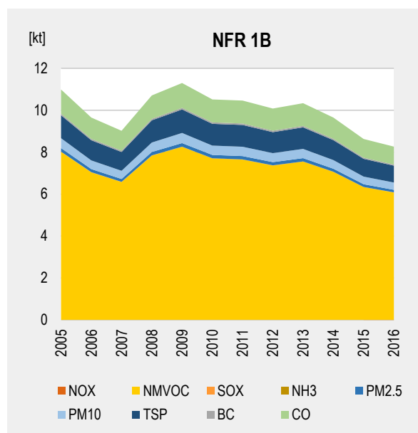
Obr. 5.7 Vývojové trendy emisií znečisťujúcich látok v sektore fugitívne emisie v rokoch 2005 – 2016
