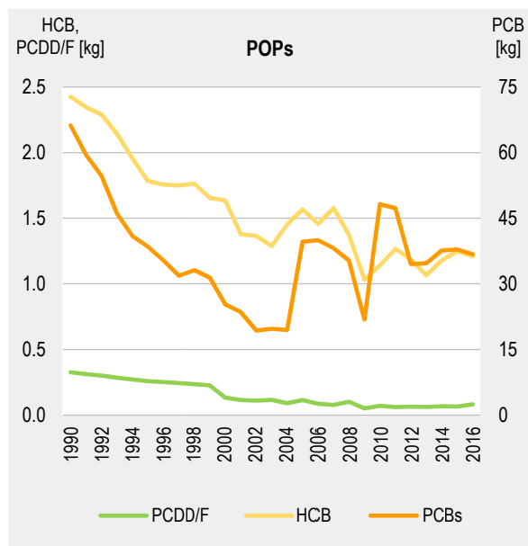
Obr. 5.4 Vývojové trendy perzistentních organických látek (POPs) v letech 1990 – 2016
