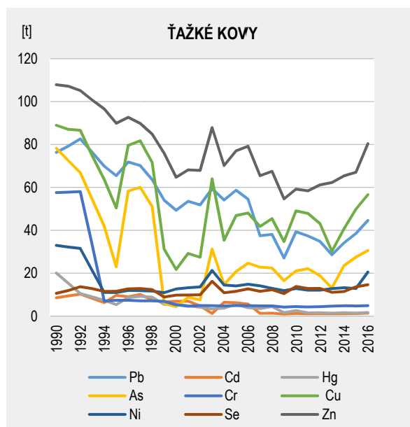
Obr. 5.2 Vývojové trendy vybraných těžkých kovů v letech 1990 – 2016
