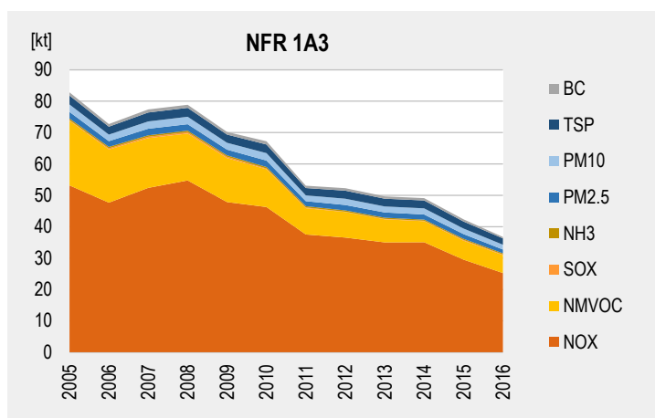
Obr. 5.8 Vývojové trendy emisií znečisťujúcich látok v sektore doprava v rokoch 2005 – 2016
