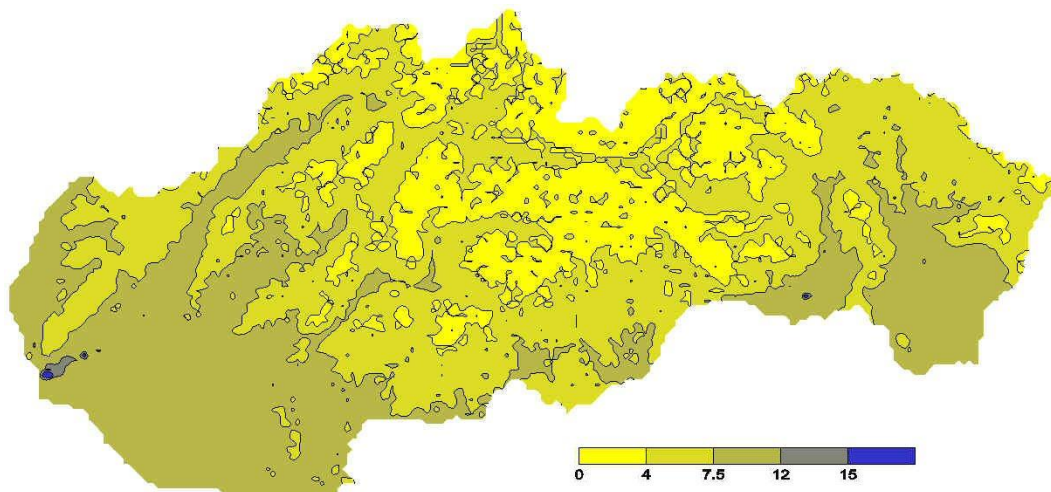
Obr. 4.4 Priemerná ročná koncentrácia \text{NO}_x ( \mu\text{g}\cdot\text{m}^{-3} ), rok 2017.
