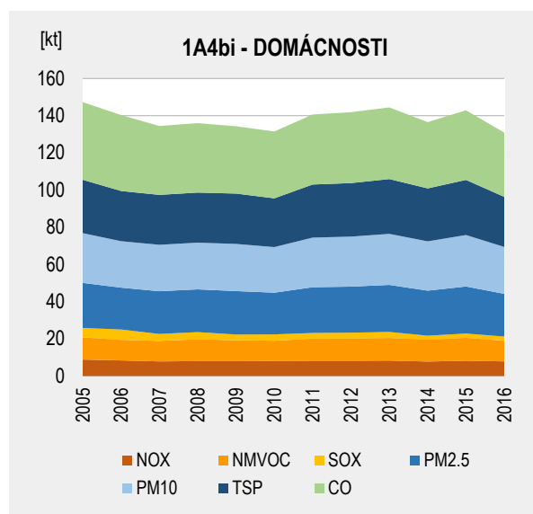
Obr. 5.9 Vývojové trendy emisií znečisťujúcich látok v sektore domácnosti v rokoch 2005–2016
