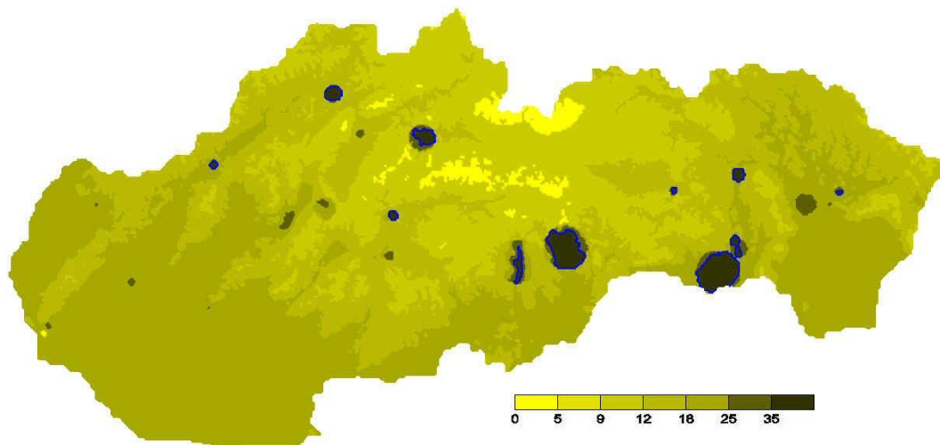
Obr. 4.13 Počet dní s prekročením limitnej hodnoty pre 24-hodinovú koncentráciu PM_{10} ( 50 \mu g \cdot m^{-3} ) v roku 2017. (Modrá čiara ohraničuje územie s prekročenou limitnou hodnotou)
