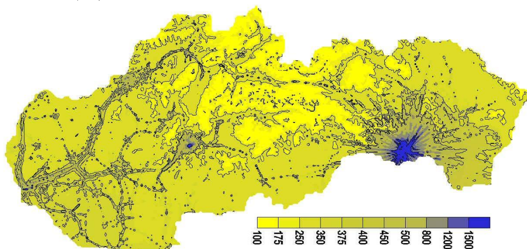
Obr. 4.7 Maximálne denné 8-hodinové klzavé priemerné koncentrácie ( \mu\text{g.m}^{-3} ) oxidu uhoľnatého (CO), rok 2017.
