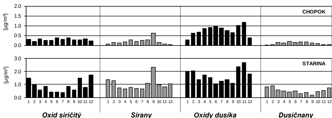
Obr. 3.1 Priemerné mesačné koncentrácie znečisťujúcich látok v ovzduší – 2017 (prepočítané na síru, resp. dusík)
