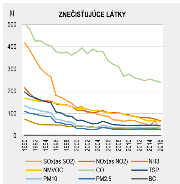
Obr. 5.1 Vývojové trendy vybraných znečišťujících látek v letech 1990 – 2016
