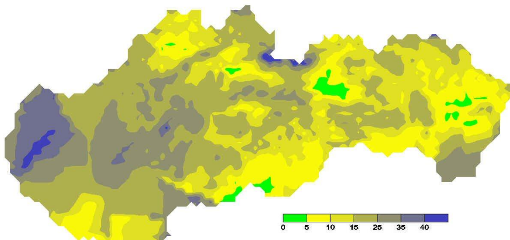
Obr. 4.10 Počet dní, v ktorých bola prekročená cieľová hodnota ozónu pre ochranu ľudského zdravia ( 120 \mu\text{g}\cdot\text{m}^{-3} ) počas rokov 2015–2017. (svetlejšia čiara ohraničuje územie s prekročenou limitnou hodnotou)
