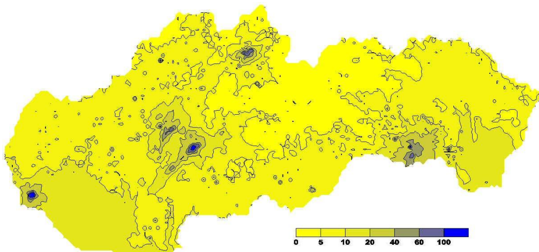
Obr. 4.3 99,7 percentil priemernej hodinovej koncentrácie \text{SO}_2 ( \mu\text{g.m}^{-3} ), rok 2017.
