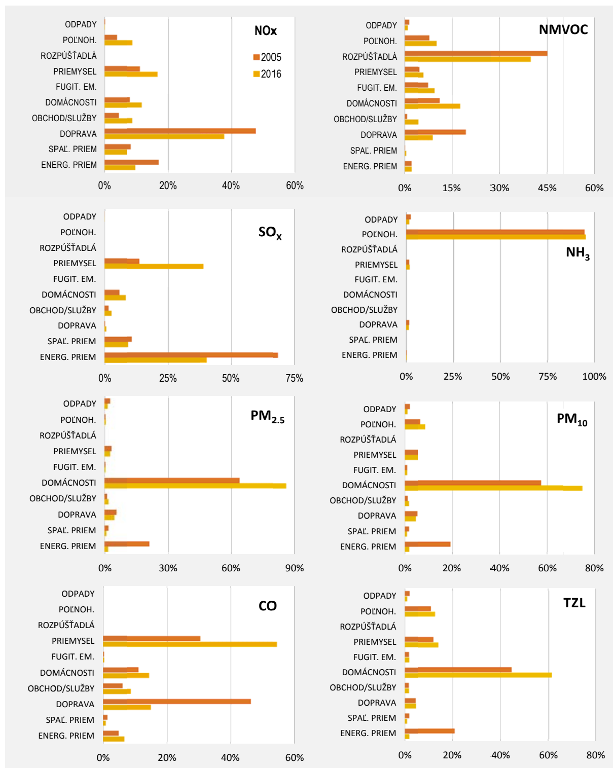
Obr. 5.5 Porovnanie emisií základného roku 2005 a emisií aktuálne dostupného roku 2016 vybraných znečisťujúcich látok \text{NO}_x , NMVOC, \text{SO}_x , \text{NH}_3 , \text{PM}_{2.5} , \text{PM}_{10} , TZL, CO v členení jednotlivých odvetví hospodárstva. Grafy uvádzajú percentuálny podiel emisií jednotlivých sektorov na celoslovenskej bilancii.
