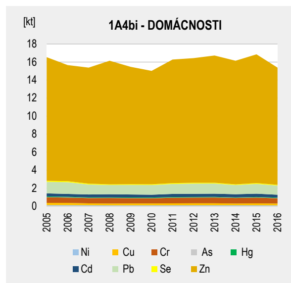
Obr. 5.10 Vývojové trendy emisií ťažkých kovov v sektore domácnosti v rokoch 2005–2016
