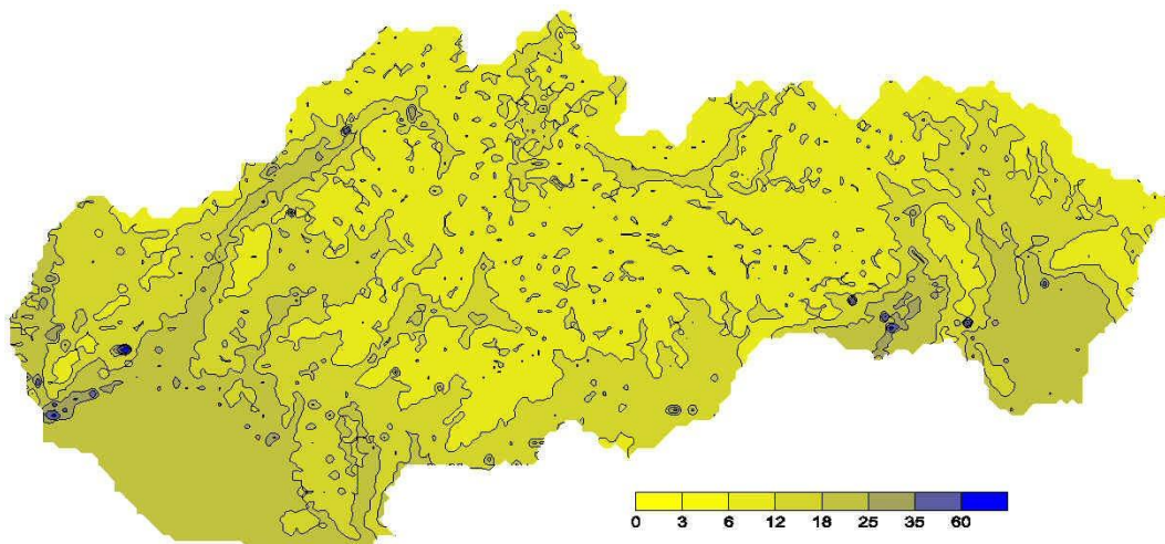
Obr. 4.6 99,8 percentil hodinovej koncentrácie \text{NO}_2 ( \mu\text{g.m}^{-3} ), rok 2017.
