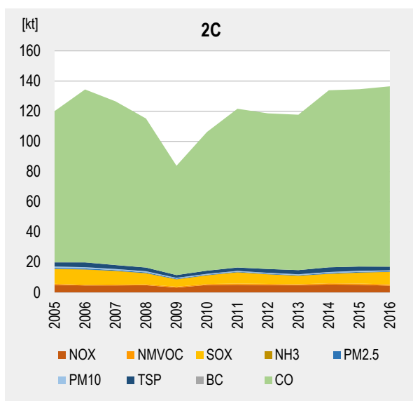
Obr. 5.13 Vývojové trendy emisií ZL v sektore výroba kovov v rokoch 2005 – 2016
