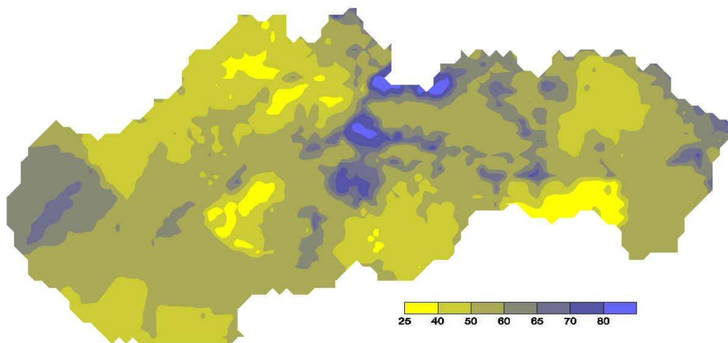
Obr. 4.9 Priemerné ročné koncentrácie prízemného ozónu (µg.m -3 ), rok 2017.
