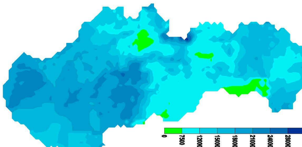
Obr. 4.11 Priemerné hodnoty AOT40 ( \mu\text{g}\cdot\text{m}^{-3}\cdot\text{h} ) za obdobie piatich rokov (2013–2017) pre ochranu vegetácie korigované na chýbajúce obdobie. (žltá čiara ohraničuje územie s prekročenou limitnou hodnotou)
