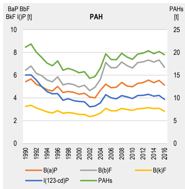
Obr. 5.3 Vývojové trendy polycyklických aromatických uhlovodíků (PAH) v letech 1990 – 2016
