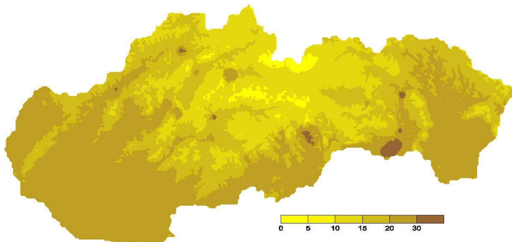
Obr. 4.12 Priemerná ročná koncentrácia PM_{10} ( \mu g \cdot m^{-3} ), rok 2017.
