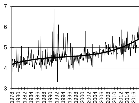
Obr. 3.2 pH v atmosférických zrážkach – Chopok
