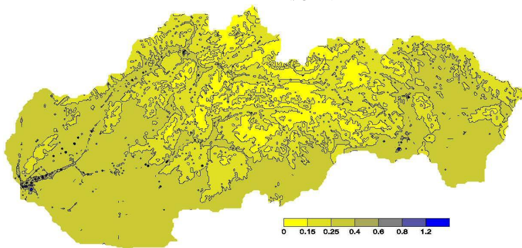
Obr. 4.8 Priemerná ročná koncentrácia benzénu ( \mu\text{g.m}^{-3} ), rok 2017.
