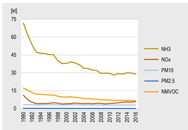
Obr. 5.15 Vývoj emisií v poľnohospodárstve
